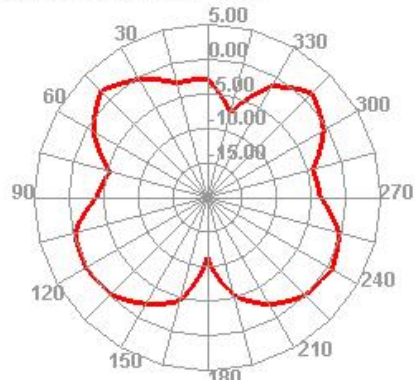
2500.000MHz E2
