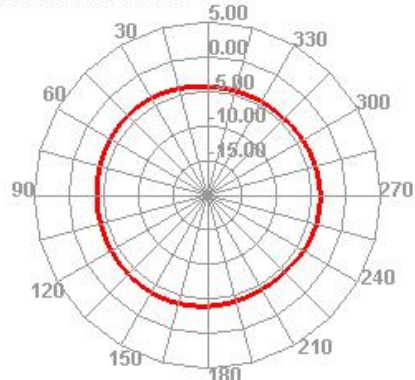
2500.000MHz H
