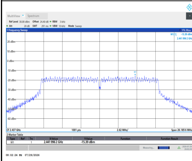
MIMO Ant. 8
