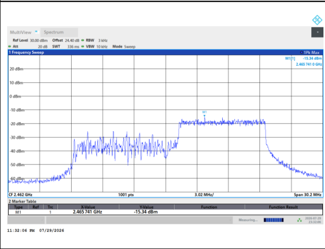
MIMO Ant. 9
