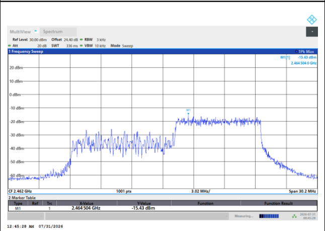
MIMO Ant. 9
