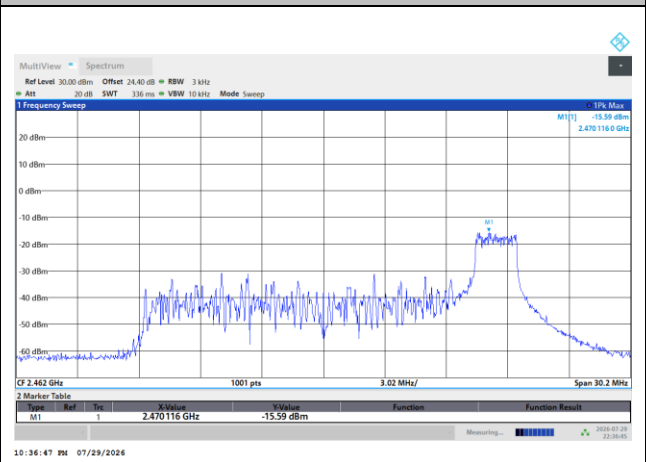
MIMO Ant. 9
