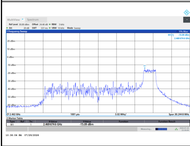
MIMO Ant. 8
