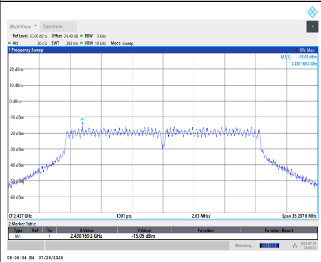
MIMO Ant. 9
