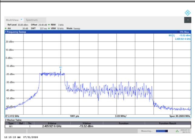
MIMO Ant. 9
