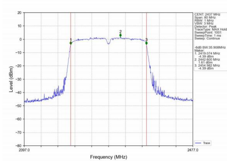
802.11n(HT40)_MCH_2437MHz_Ant1 (SISO)_NTNV
