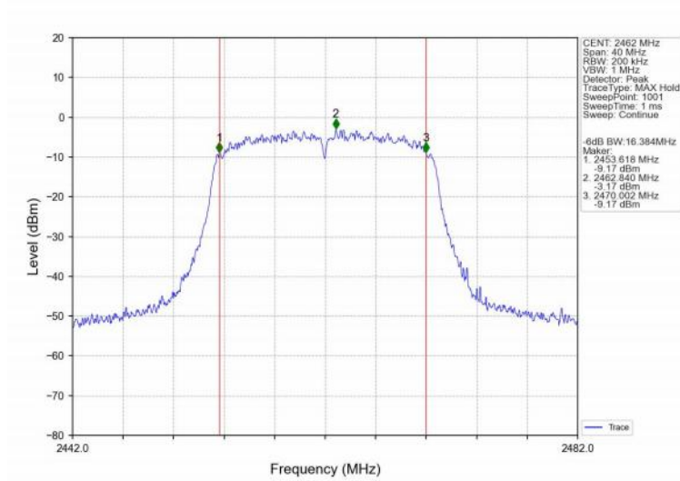
802.11n(HT20)_HCH_2462MHz_Ant1 (SISO)_NTNV
