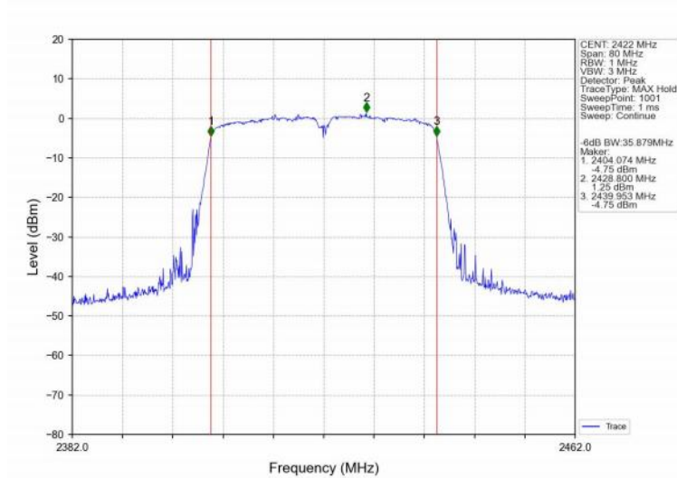
802.11n(HT40)_LCH_2422MHz_Ant1 (SISO)_NTNV
