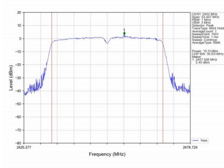
802.11n(HT40)_HCH_2452MHz_Ant1 (SISO)_NTNV
