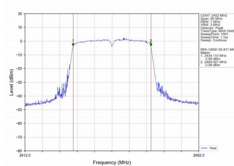
802.11n(HT40)_HCH_2452MHz_Ant1 (SISO)_NTNV
