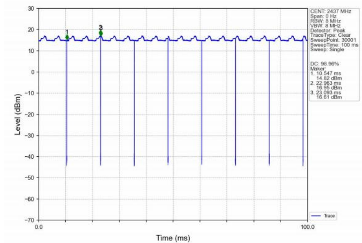
802.11b_MCH_2437MHz_Ant1 (SISO)_NTNV
