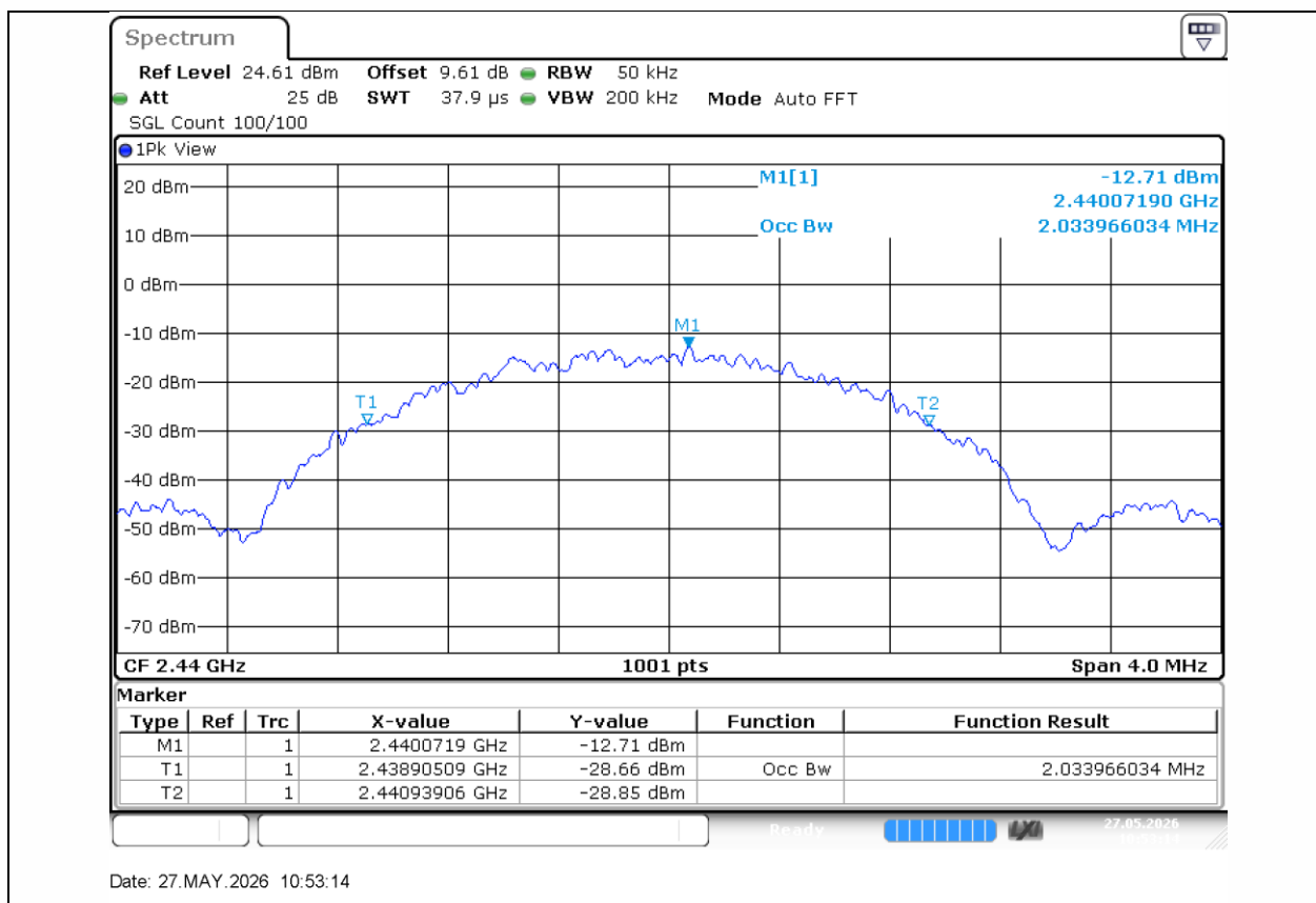
BLE_2M-Ant1-2440
