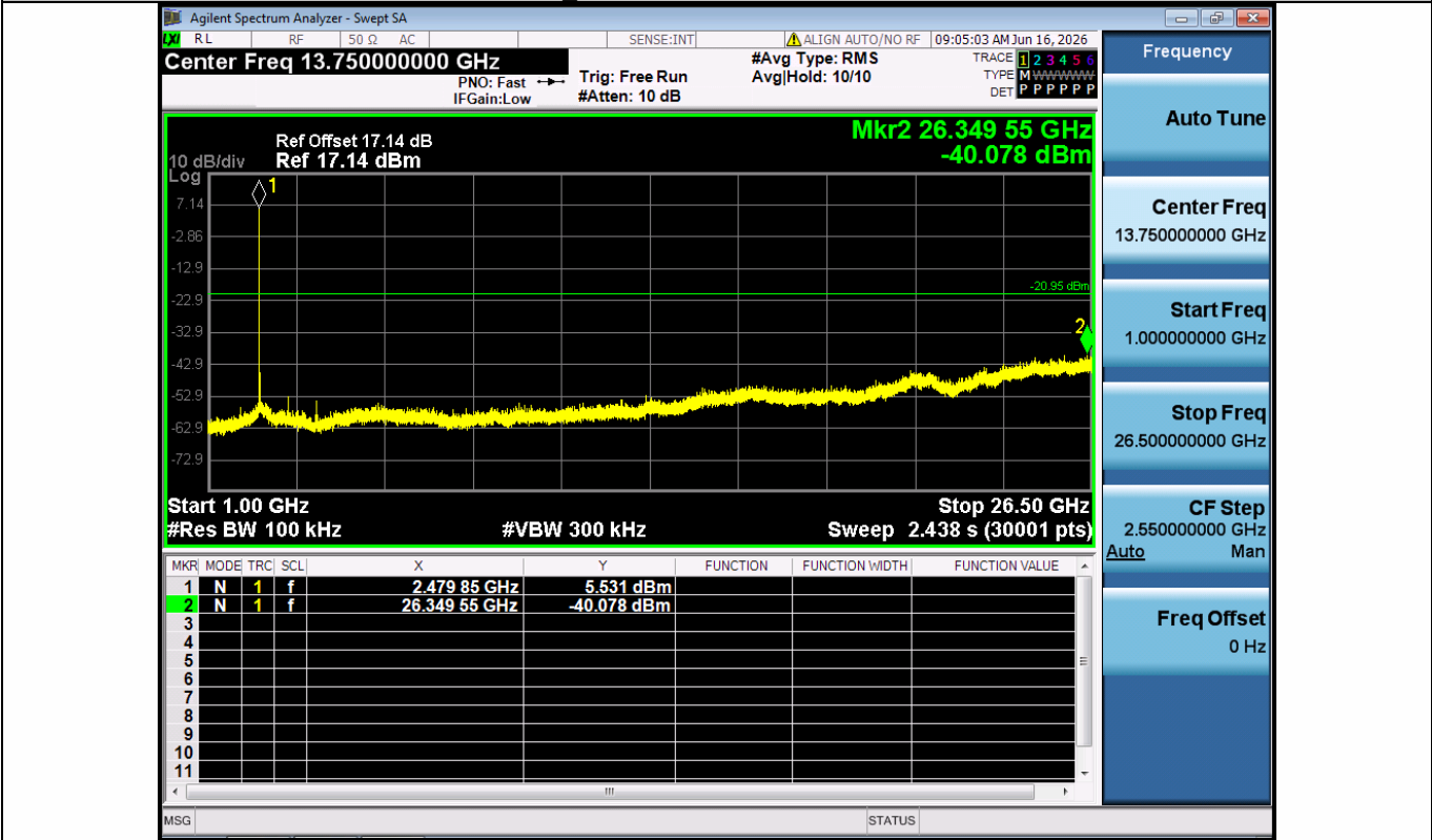
BLE 2M-Ant1-2480-1000~26500-PASS
