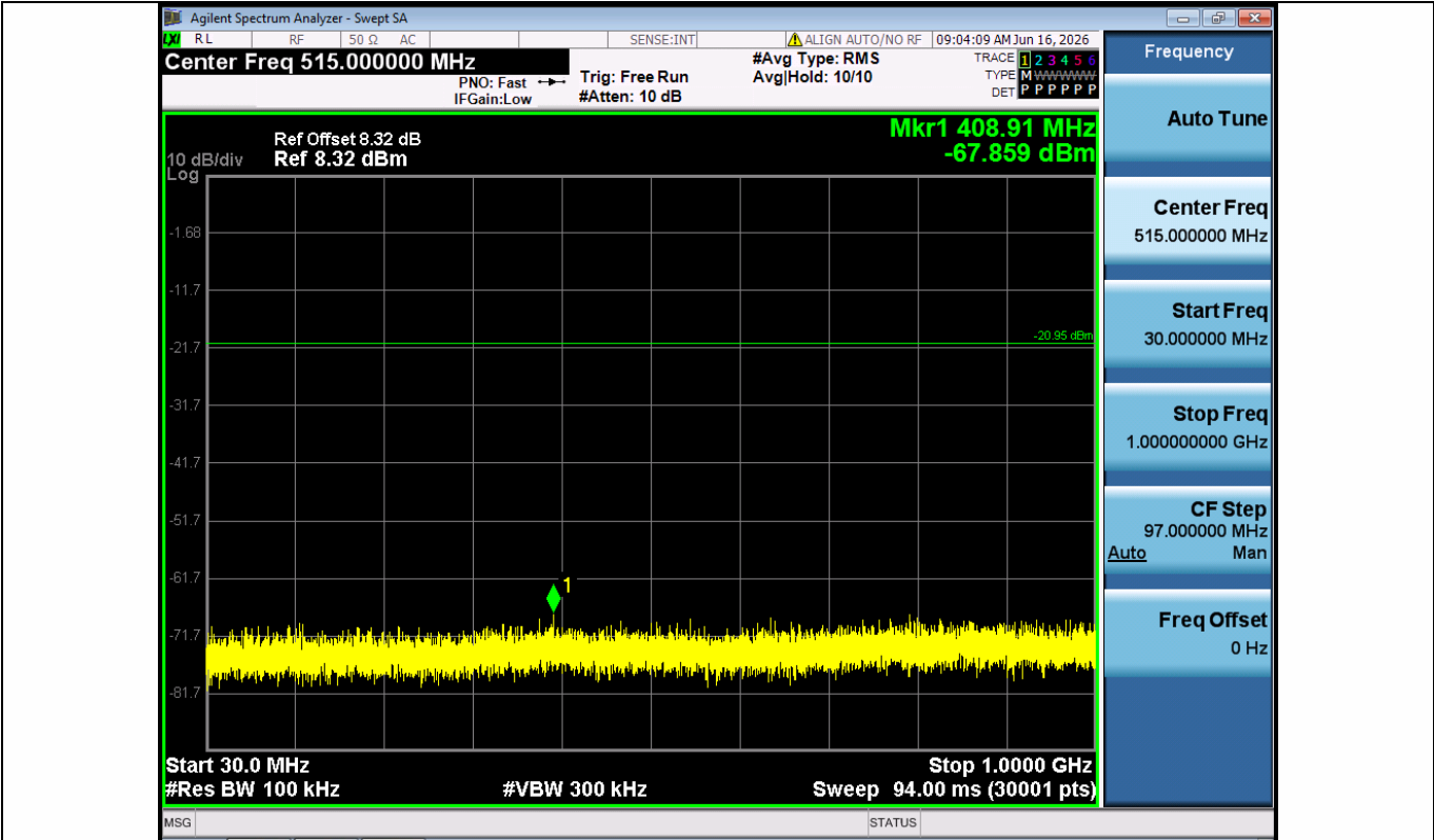
BLE 2M-Ant1-2480-30~1000-PASS
