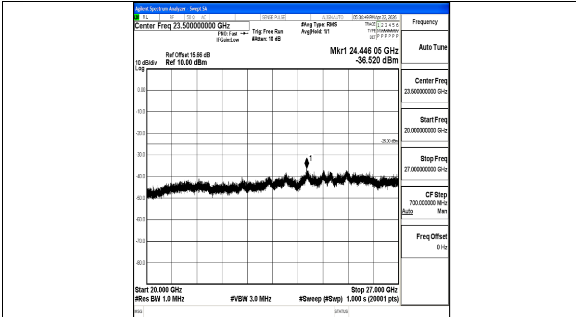
Band7_20MHz_QPSK_20850_1RB#0_20000~27000_20000~27000
