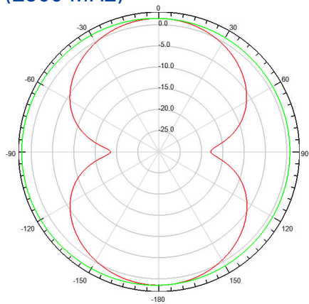
2D 增益模式 2D Gain Pattern (2500 MHz)
