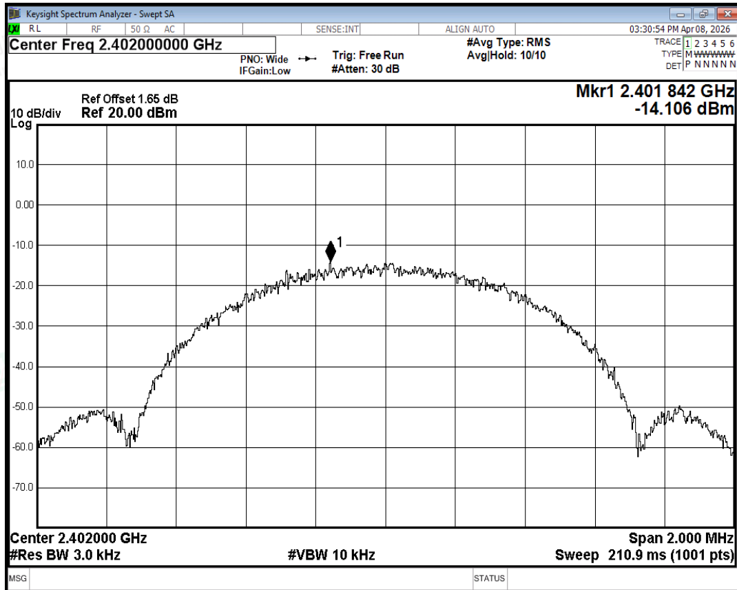
PSD NVNT BLE 2402MHz Ant1
