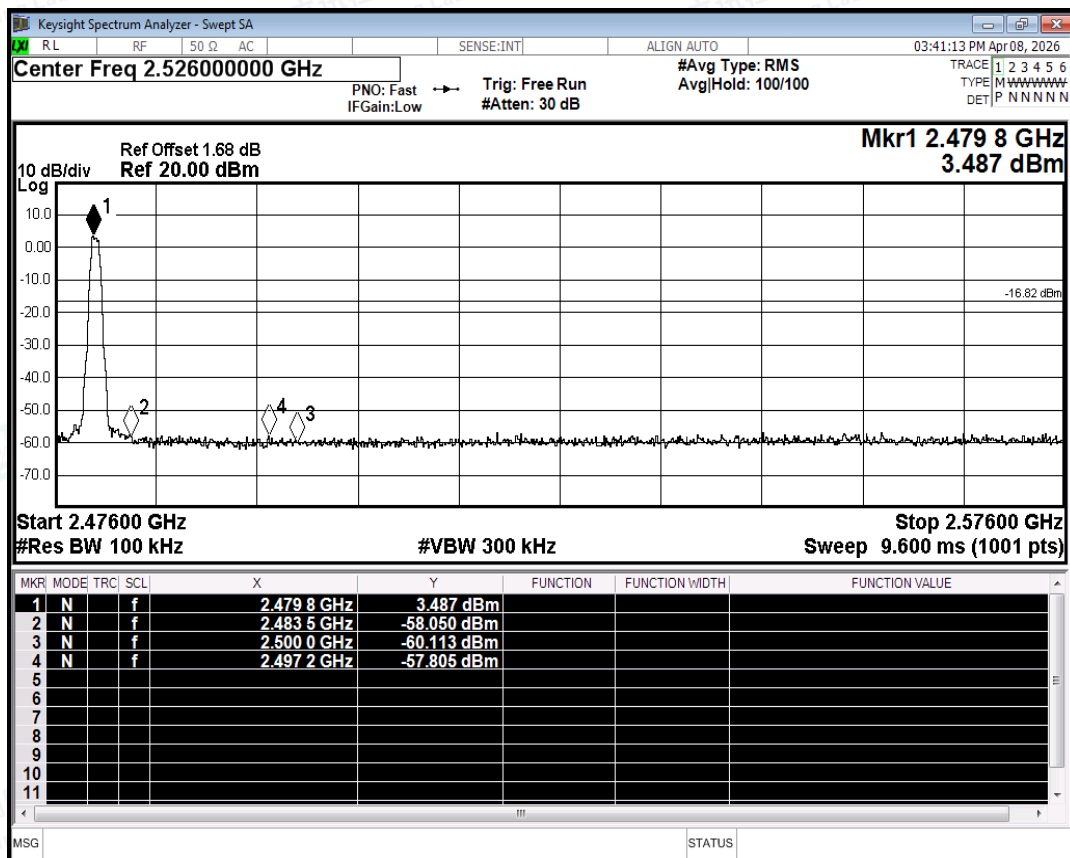
Band Edge NVNT BLE 2480MHz Ant1 Emission
