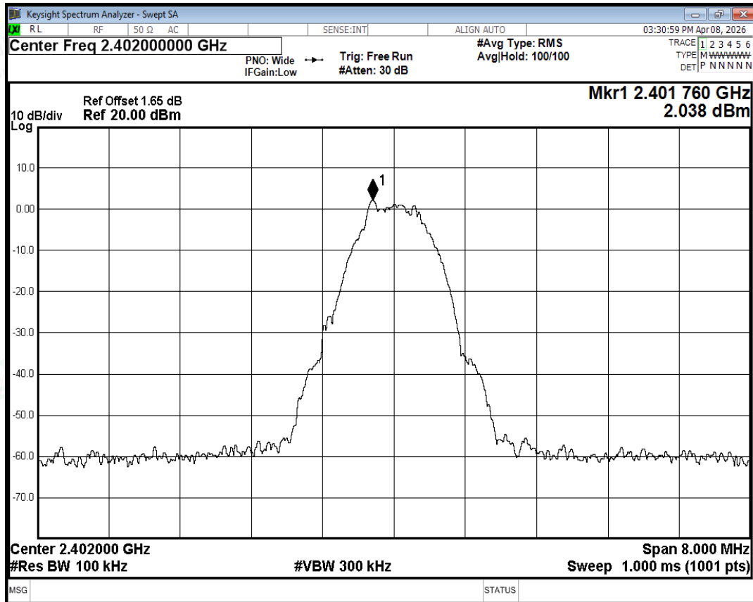
Band Edge NVNT BLE 2402MHz Ant1 Ref
