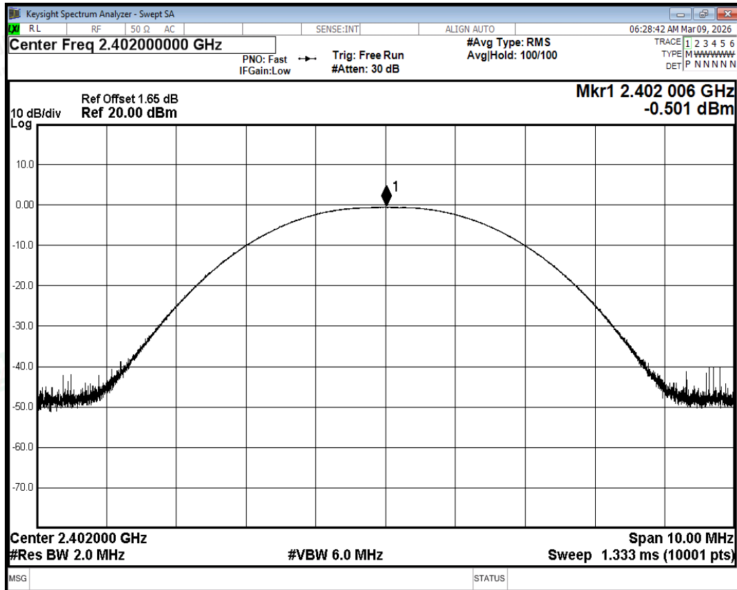
Peak Power NVNT BLE 2402MHz Ant1
