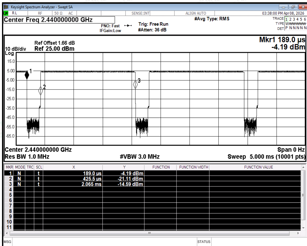
Duty Cycle NVNT BLE 2440MHz Ant1
