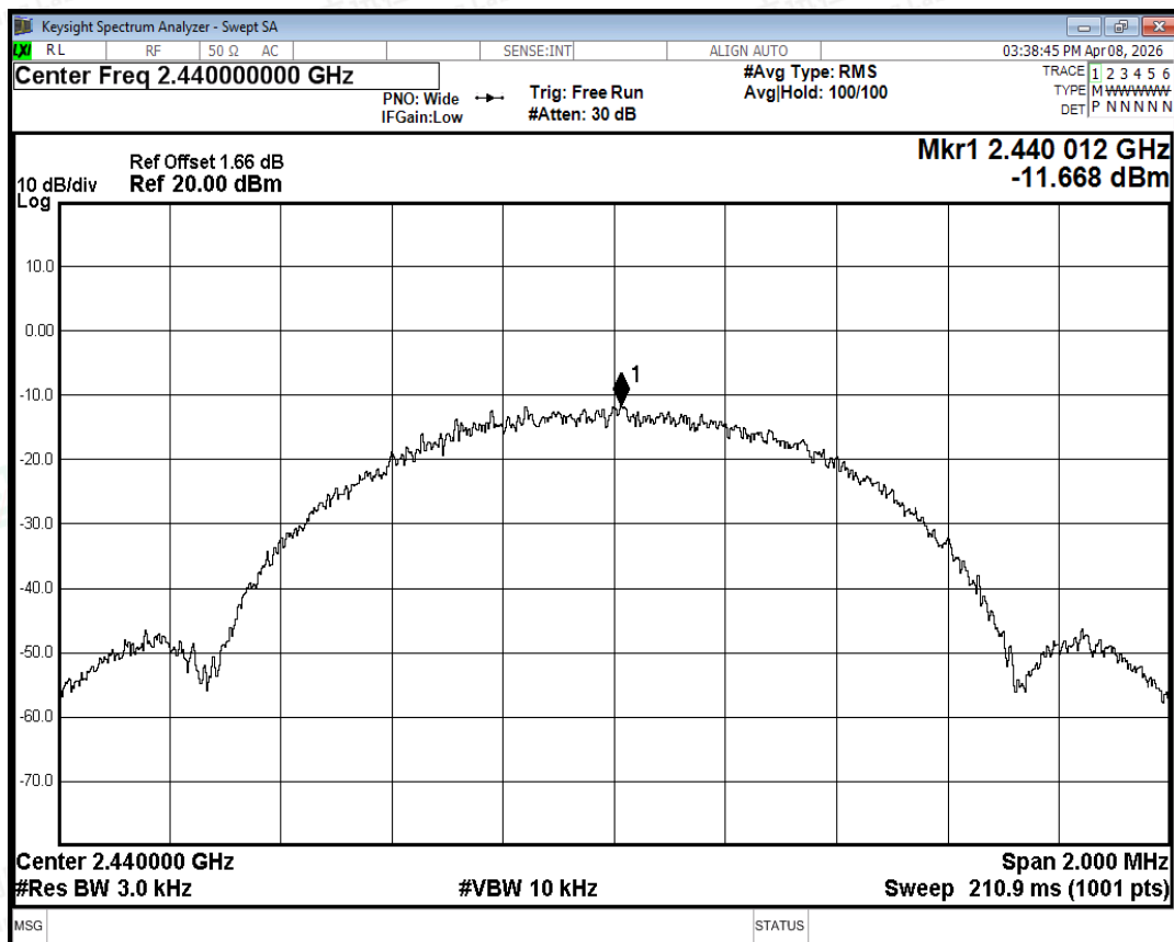
PSD NVNT BLE 2440MHz Ant1
