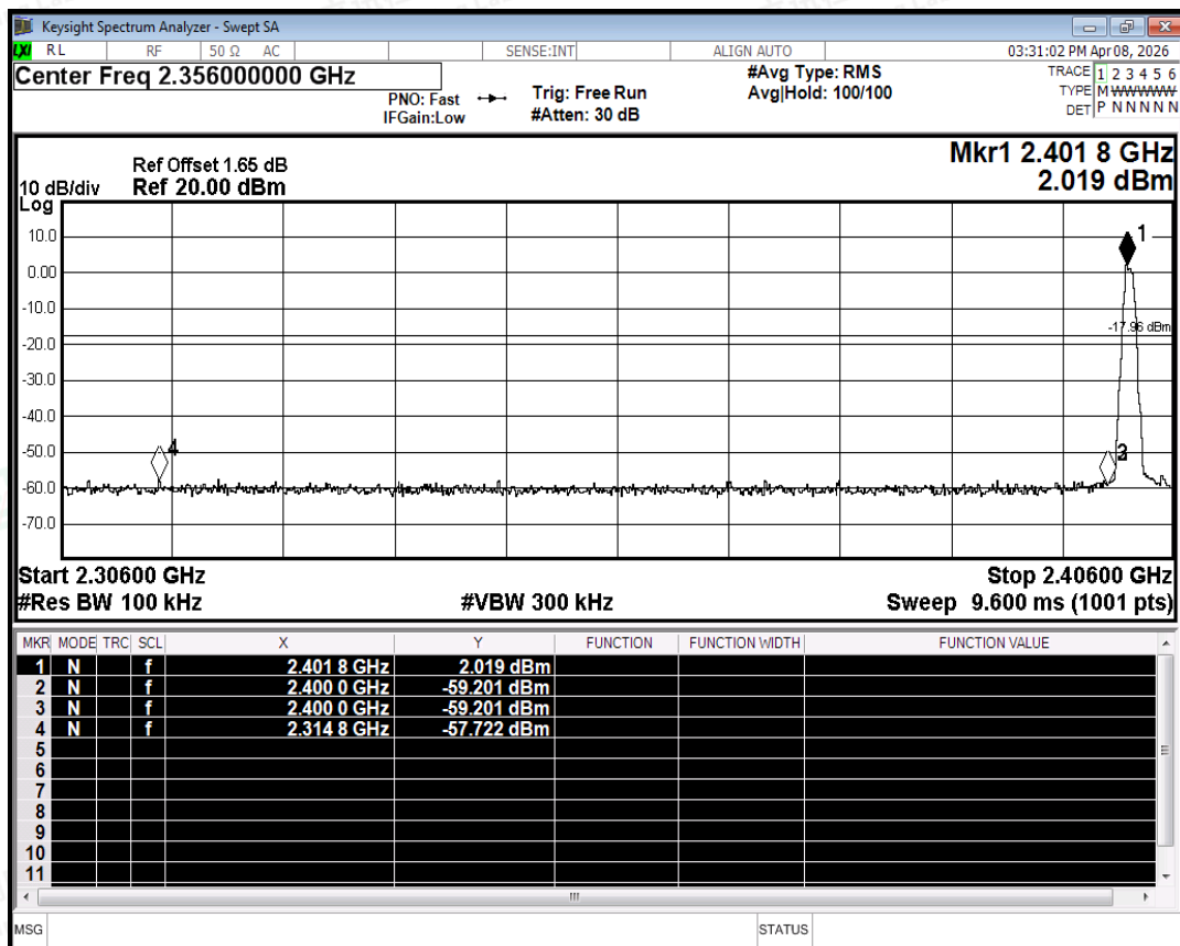
Band Edge NVNT BLE 2402MHz Ant1 Emission
