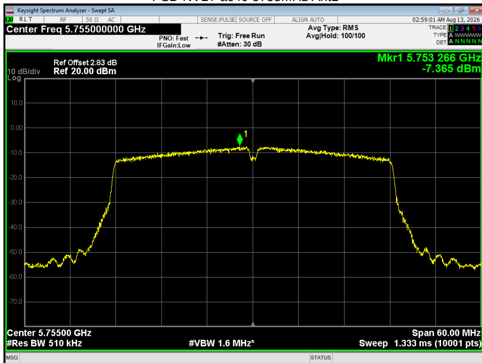
PSD NVLT ac40 5755MHz Ant1
