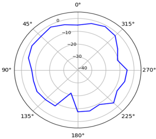
XY-Plane 2437 MHz
