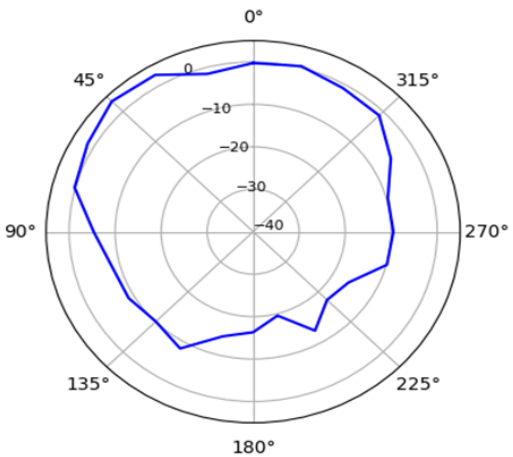
XZ-Plane 2483 MHz
