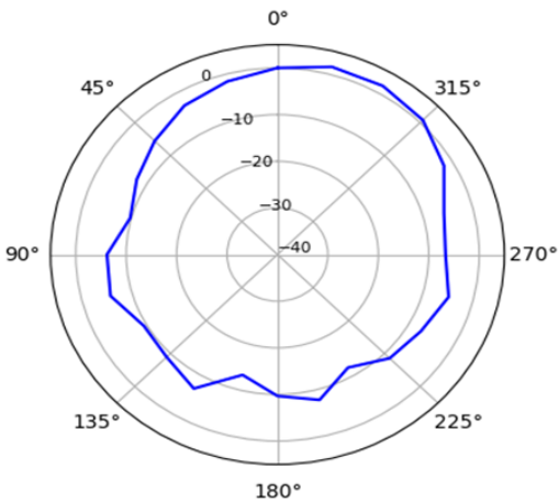
YZ-Plane 2500 MHz
