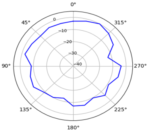
XY-Plane 2412 MHz
