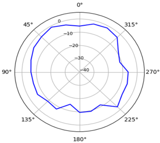
XY-Plane 2483 MHz
