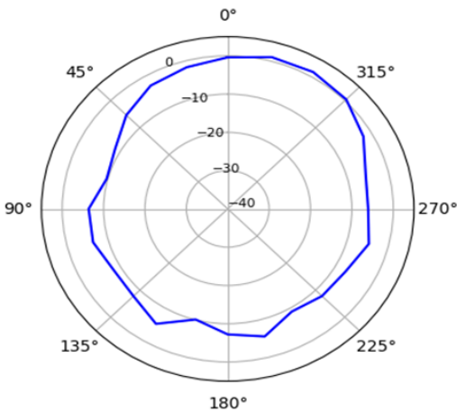
YZ-Plane 2462 MHz
