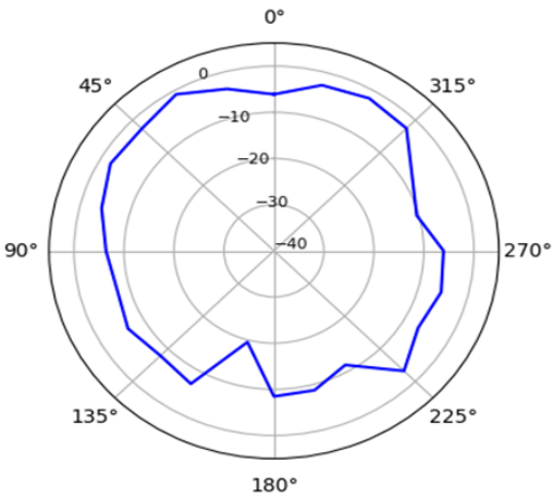
XY-Plane 2462 MHz
