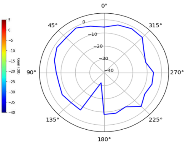
XY-Plane 2450 MHz
