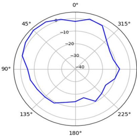
XZ-Plane 2437 MHz
