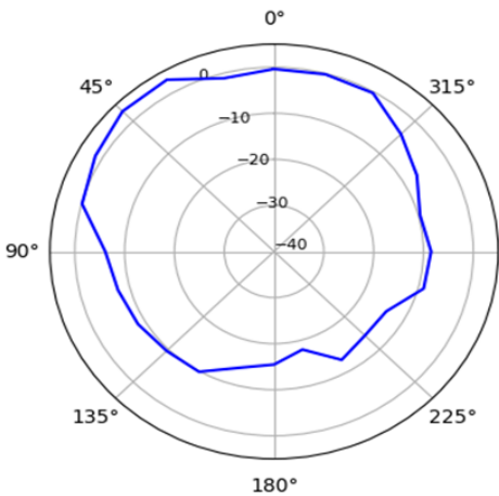
XZ-Plane 2462 MHz
