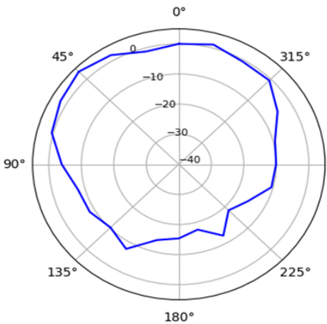
XZ-Plane 2500 MHz
