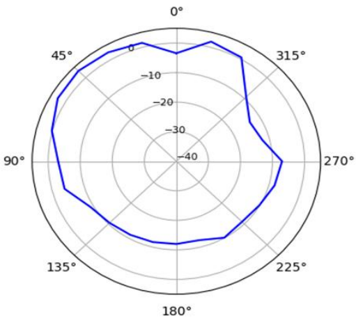
XZ-Plane 2412 MHz
