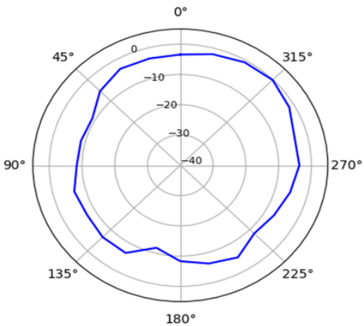
YZ-Plane 2412 MHz
