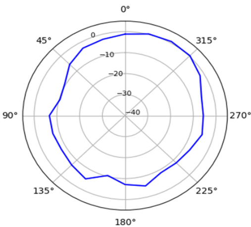
YZ-Plane 2450 MHz
