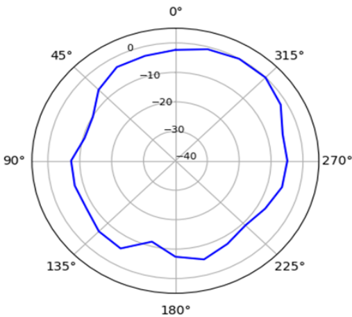
YZ-Plane 2437 MHz
