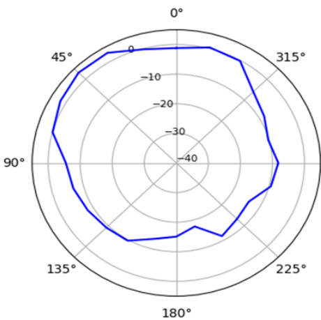
XZ-Plane 2450 MHz
