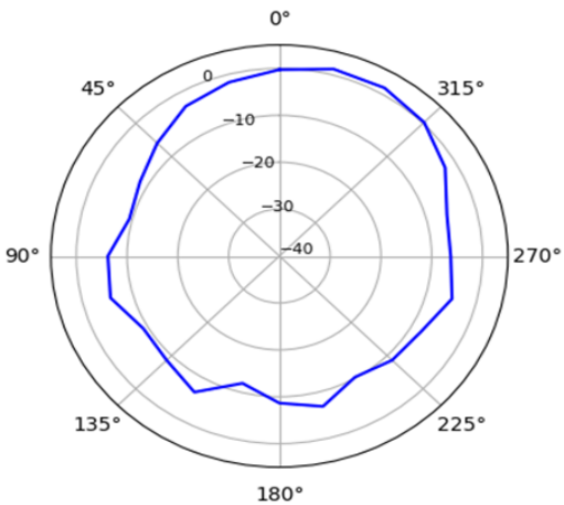
YZ-Plane 2483 MHz
