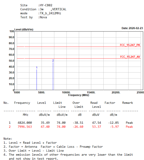
TX_b_2412MHz_V
