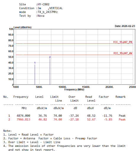
TX_b_2437MHz_V
