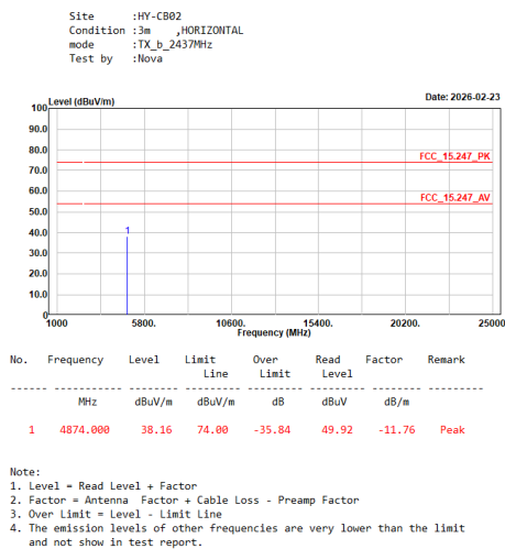
TX_b_2437MHz_H
