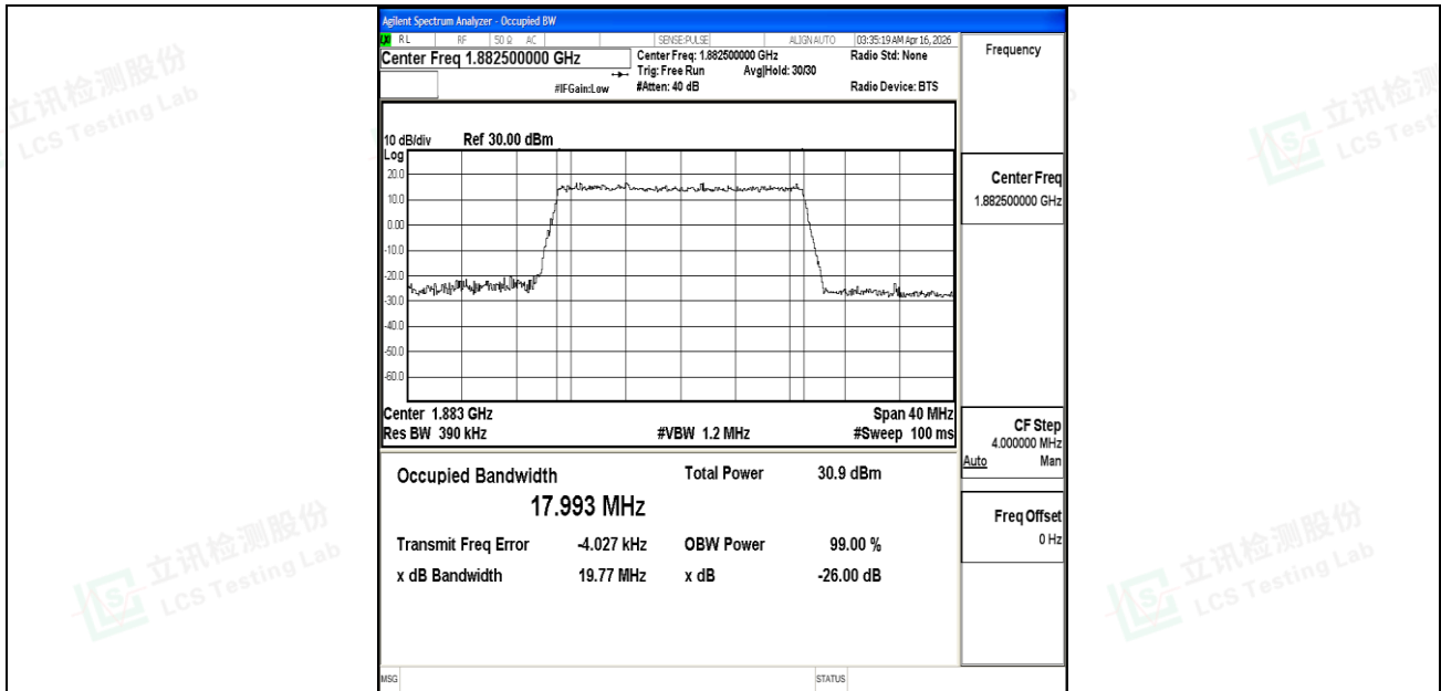
Band25-20MHz-QPSK-26365-100RB#0-PASS
