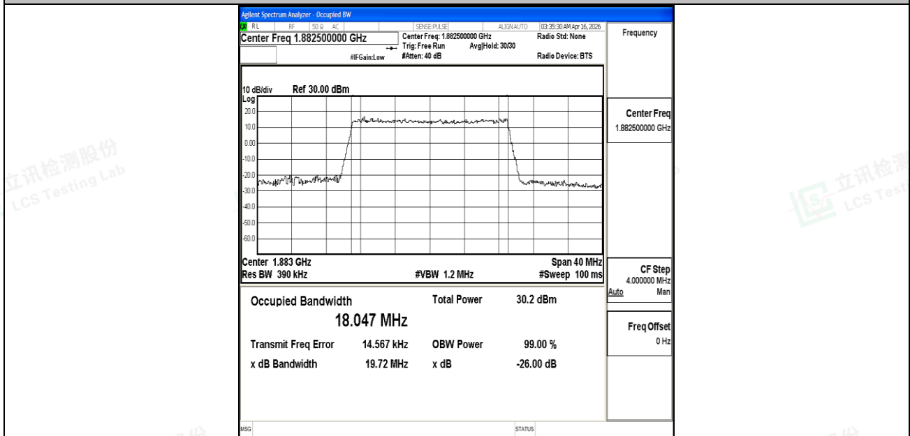
Band25-20MHz-16QAM-26365-100RB#0-PASS
