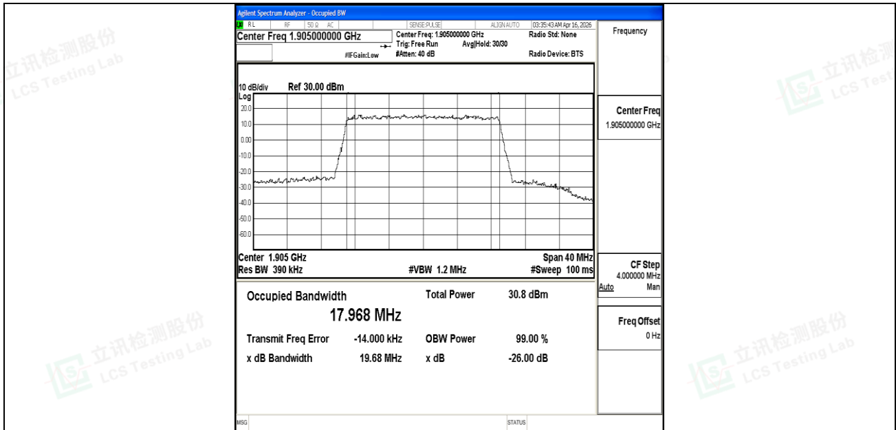
Band25-20MHz-QPSK-26590-100RB#0-PASS
