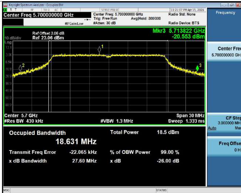
-26dB Bandwidth NVNT n20 5700MHz Ant1
