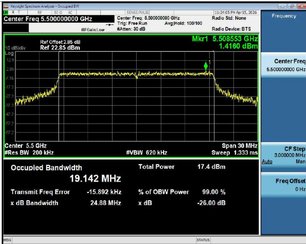
OBW NVNT ax20 5500MHz Ant1
