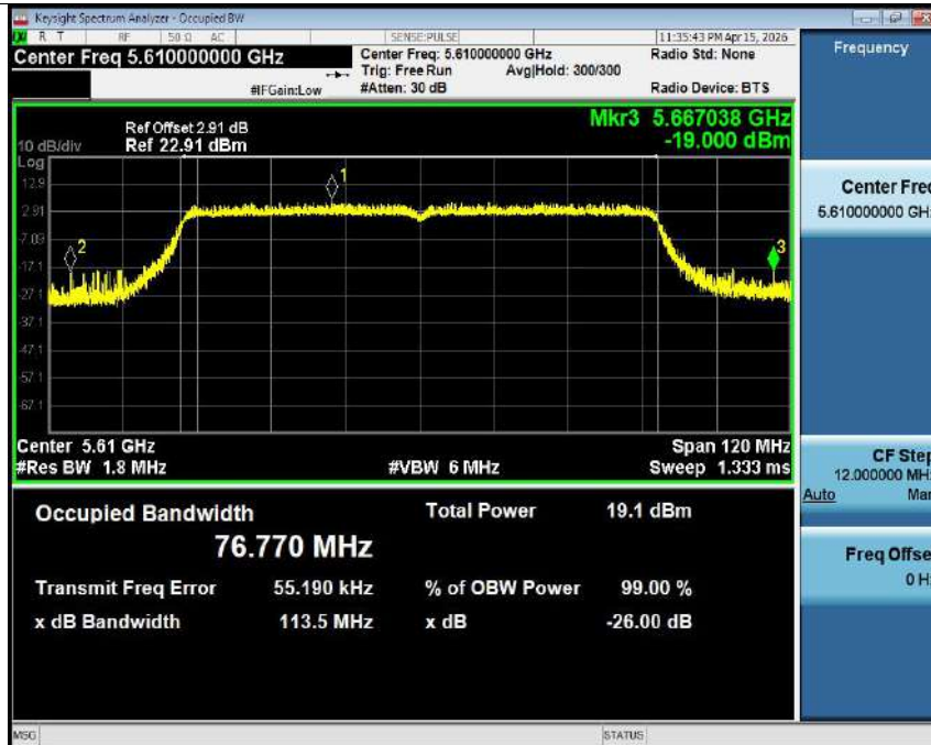
-26dB Bandwidth NVNT ac80 5610MHz Ant1
