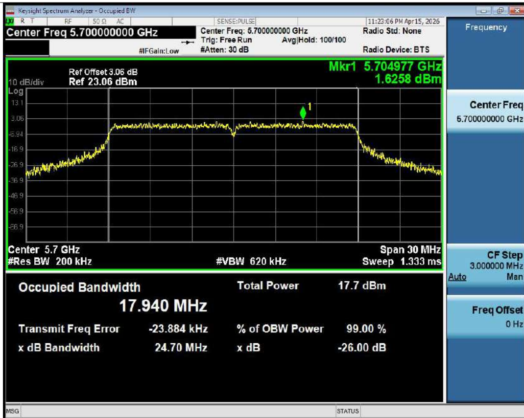
OBW NVNT ac20 5700MHz Ant1
