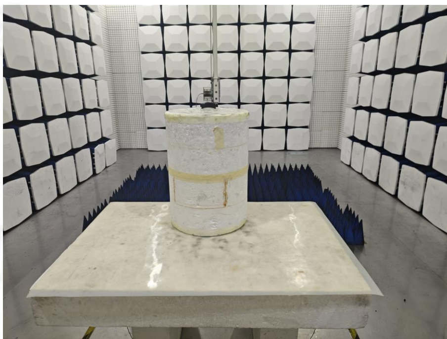
RE (1GHz-18GHz)
