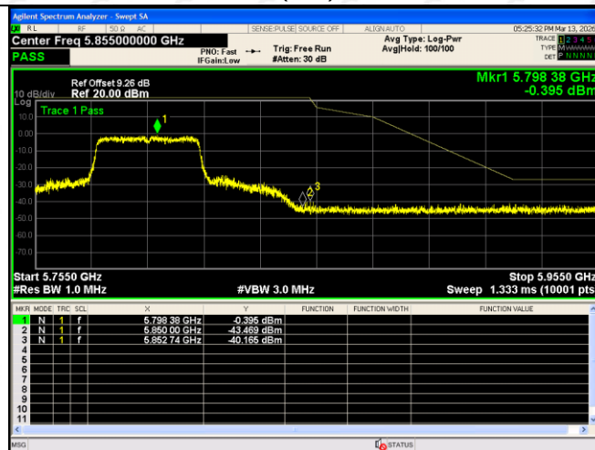
802.11(n40)-5795
