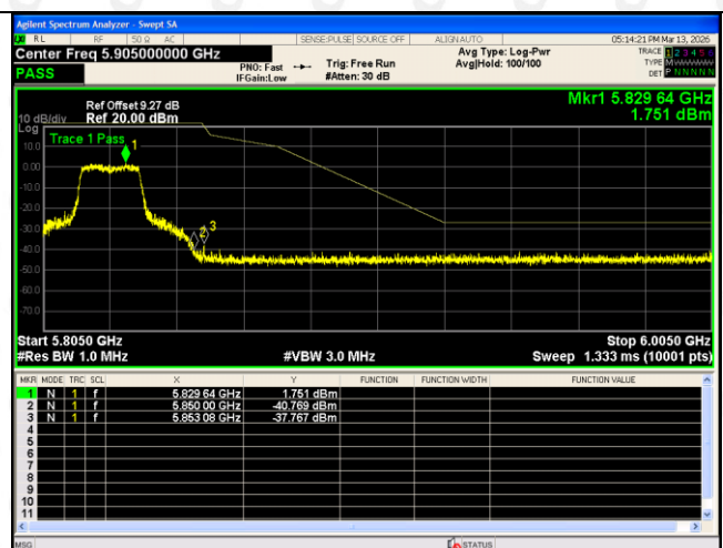
802.11(n40)-5795
