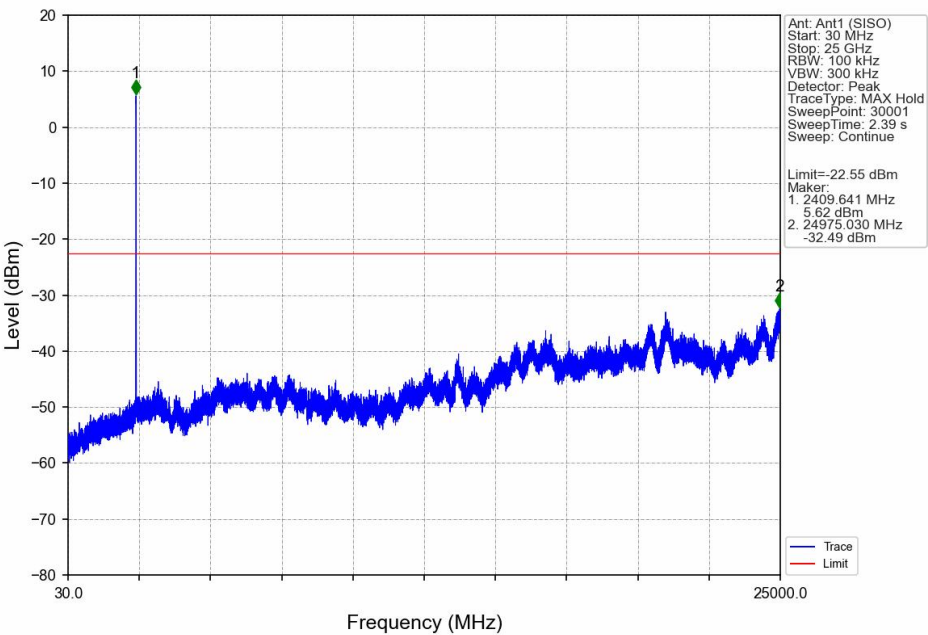
802.11b_LCH_2412MHz_Ant1 (SISO)_NTNV
