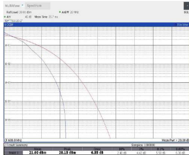
Band71-20MHz-QPSK-133372-100RB#0
