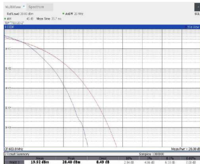
Band71-20MHz-16QAM-133372-1RB#0
