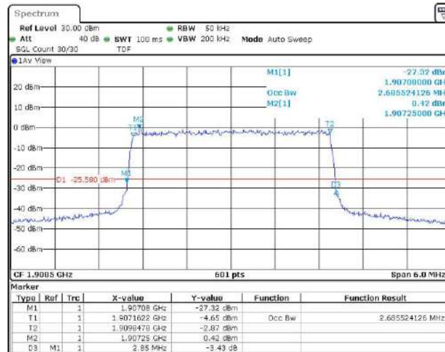
Band2-3MHz-16QAM-18615-15RB#0
