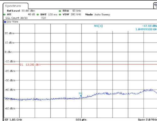
Band2-3MHz-QPSK-18615-1RB#14
