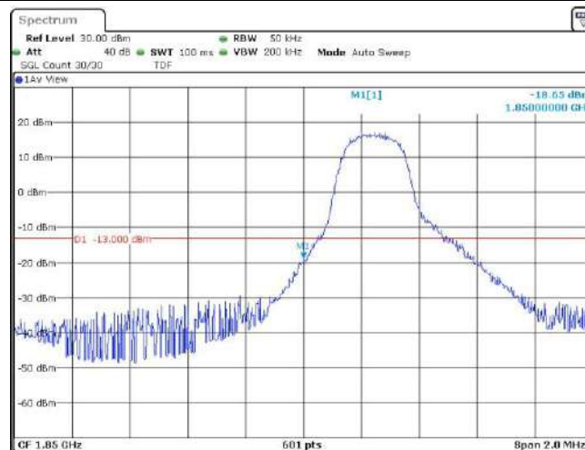
Band2-3MHz-QPSK-18615-1RB#0
