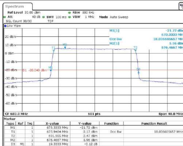
Band71-20MHz-QPSK-133372-100RB#0
