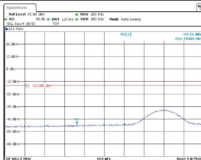
Band71-10MHz-QPSK-133172-50RB#0
