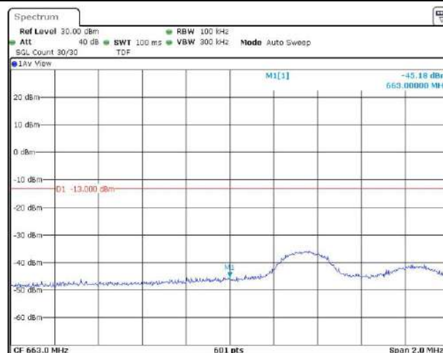
Band71-5MHz-QPSK-133147-25RB#0
