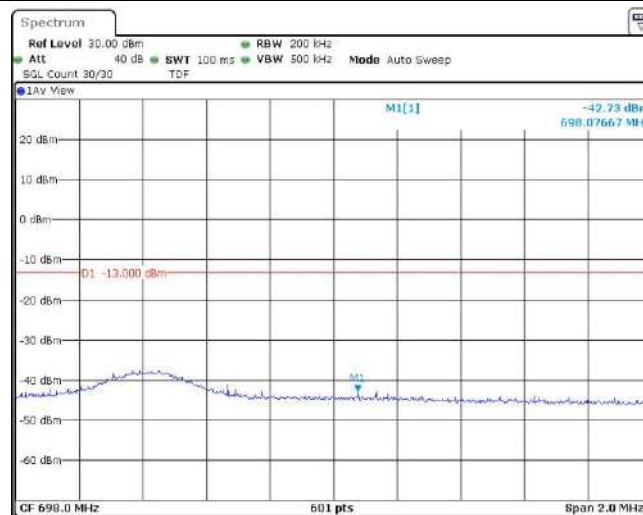
Band71-10MHz-QPSK-133422-1RB#49
