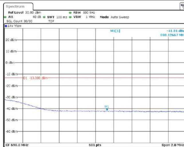
Band71-20MHz-16QAM-133372-1RB#99
