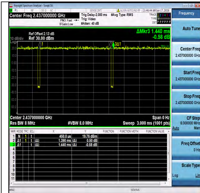
NTNV-11g-Ant1-2437
