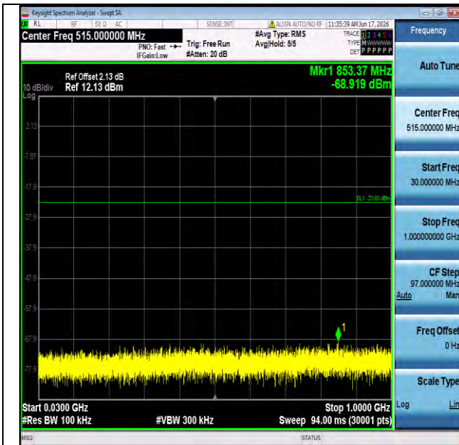
11g-Ant1-2412-30~1000-PASS
