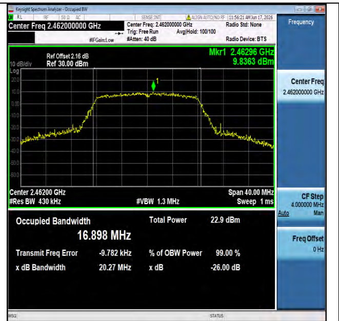
11g-Ant1-2462
