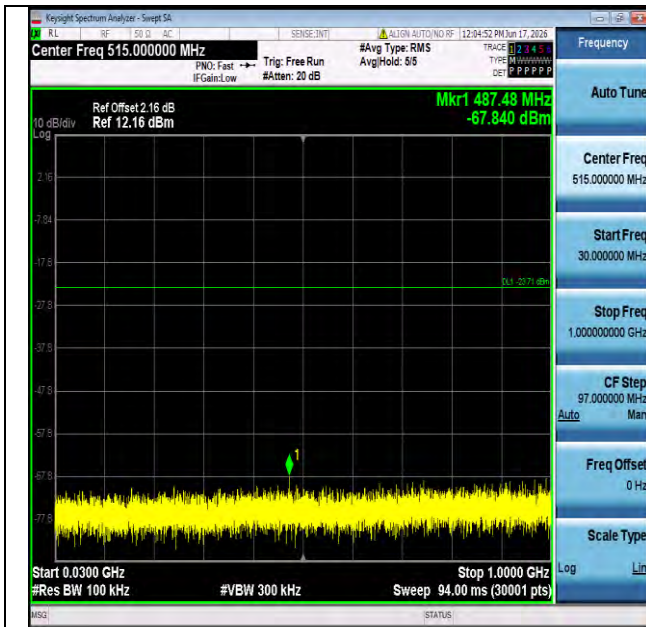
11g-Ant1-2462-30~1000-PASS
