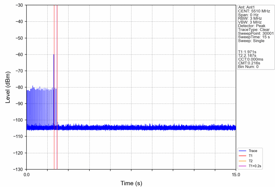
802.11n40 channel 102 5510MHz
