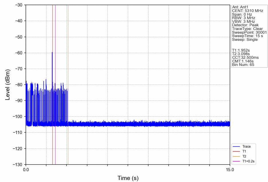
802.11n40 channel 62 5310MHz
