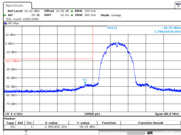
802.11b_2412MHz
