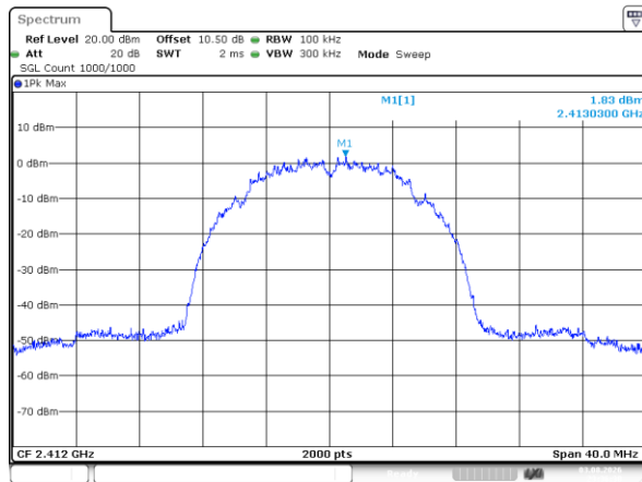
802.11b_2412MHz
