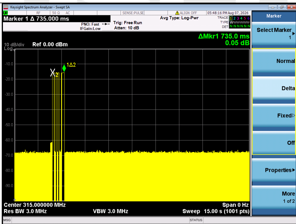
Test Plot-- TX-315M-FSK
