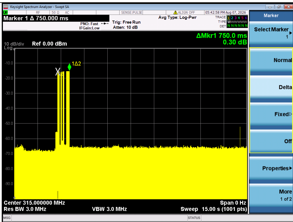
Test Plot-- TX-315M-ASK
