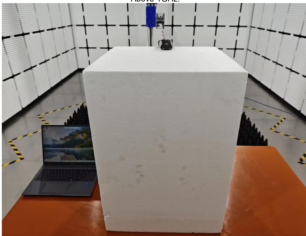
Above 1GHz:
