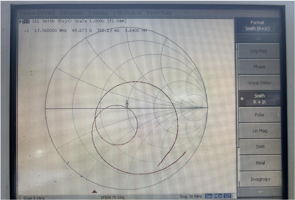
史密斯图
