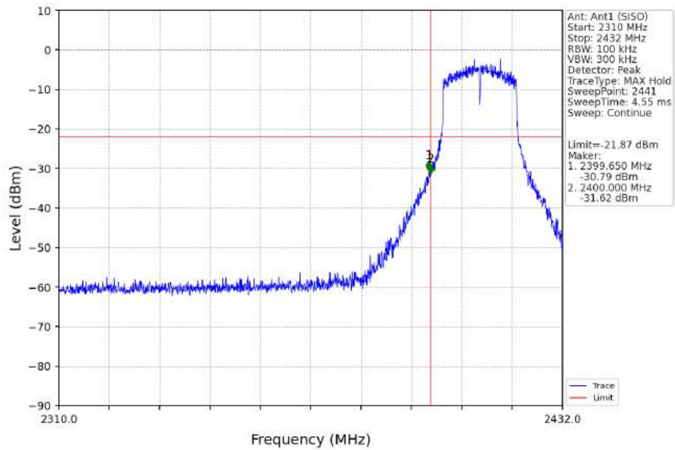
802.11n(HT20)_LCH_2412MHz_Ant1 (SISO)_NTNV
