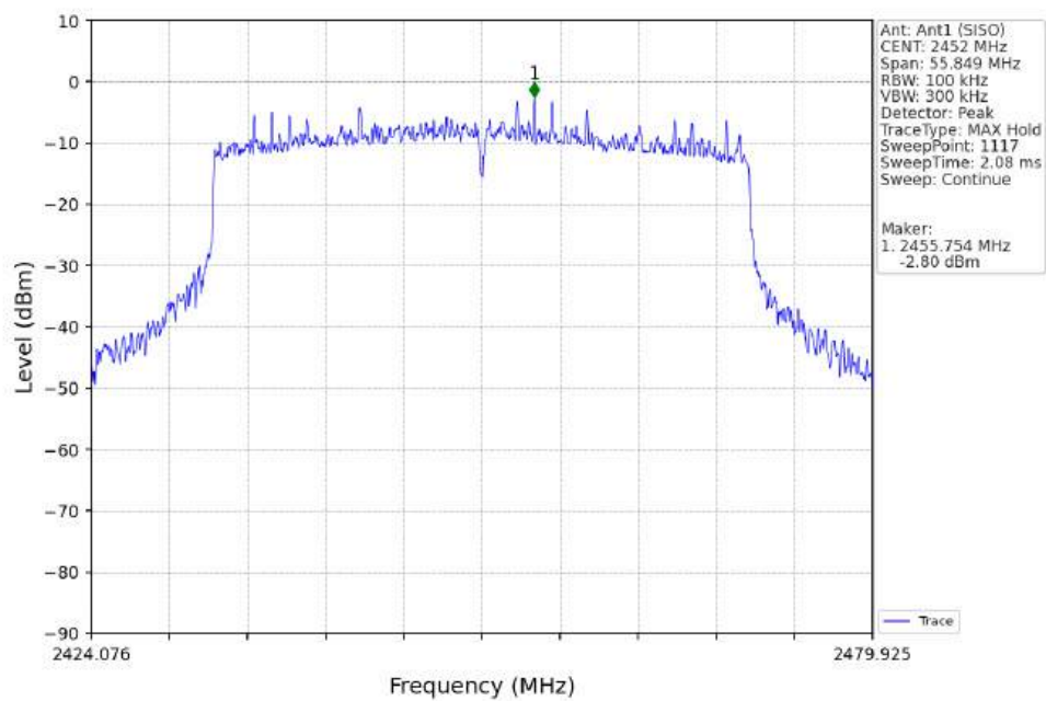
802.11ax(HEW40)_HCH_2452MHz_SU_/_Ant1 (SISO)_NTNV
