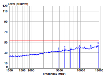
11b_TX_CH_01_Vertical-Avg
