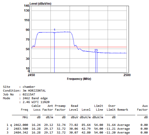
11n_HT(20M)_TX_CH_11_Horizontal-Avg
