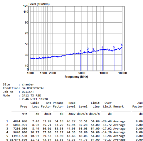
11n_HT(20M)_TX_CH_01_Horizontal-Avg
