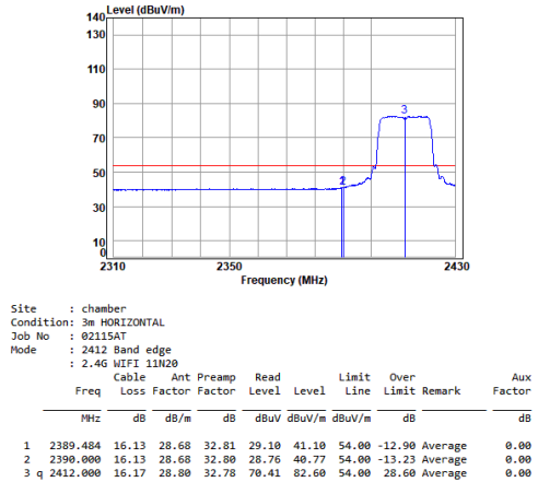
11n_HT(20M)_TX_CH_01_Horizontal-Avg
