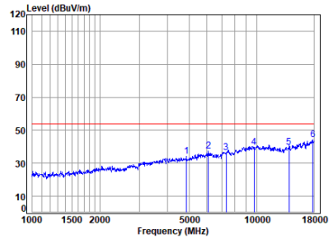
11b_TX_CH_06_Horizontal-Avg
