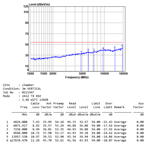
11n_HT(20M)_TX_CH_01_Vertical-Avg
