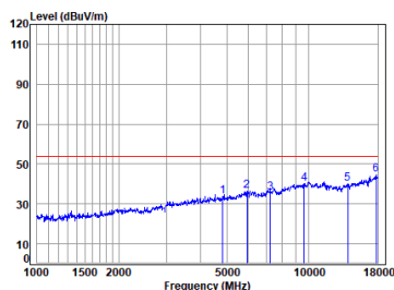
11b_TX_CH_01_Horizontal-Avg
