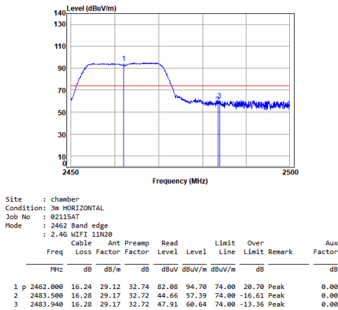
11n_HT(20M)_TX_CH_11_Horizontal-Peak
