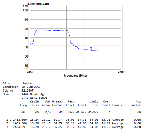
11n_HT(20M)_TX_CH_11_Vertical-Avg
