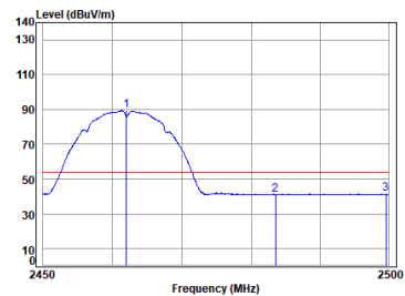
11b_TX_CH_11_Vertical-Avg
