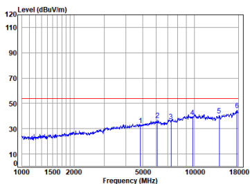
11n_HT(20M)_TX_CH_06_Horizontal-Avg
