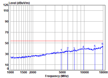
11b_TX_CH_06_Vertical-Avg
