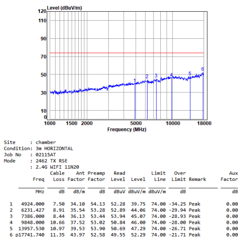
11n_HT(20M)_TX_CH_11_Horizontal-Peak
