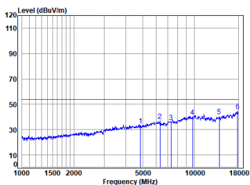
11n_HT(20M)_TX_CH_06_Vertical-Avg
