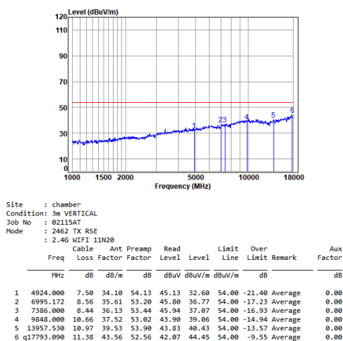
11n_HT(20M)_TX_CH_11_Vertical-Avg
