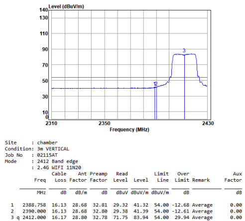
11n_HT(20M)_TX_CH_01_Vertical-Avg
