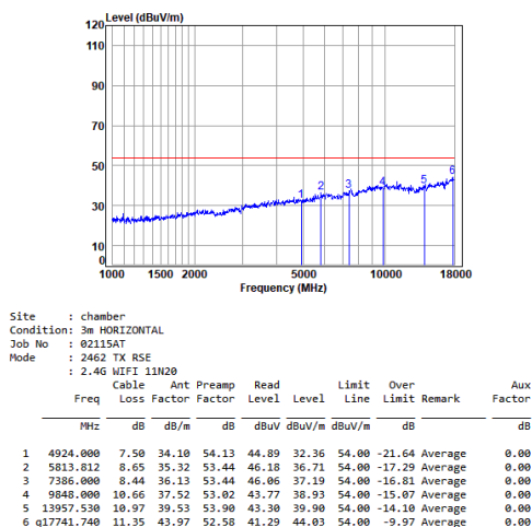
11n_HT(20M)_TX_CH_11_Horizontal-Avg
