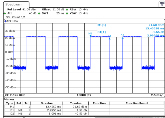
20MHz_Middle_QPSK_100@0
