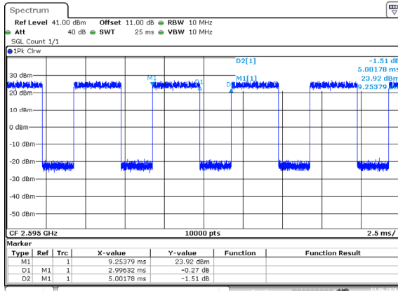
5MHz_Middle_QPSK_25@0
