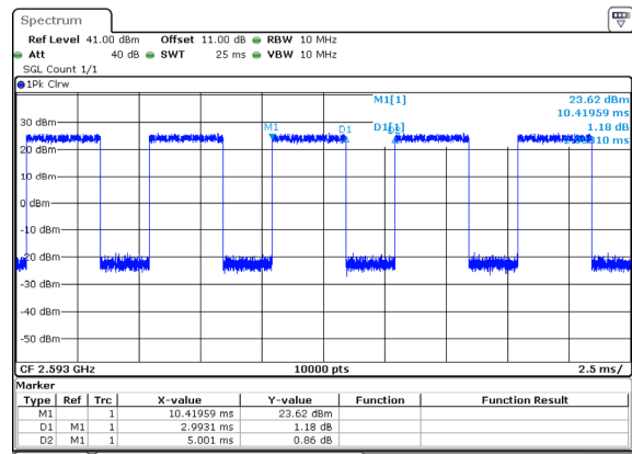
10MHz_Middle_QPSK_50@0
