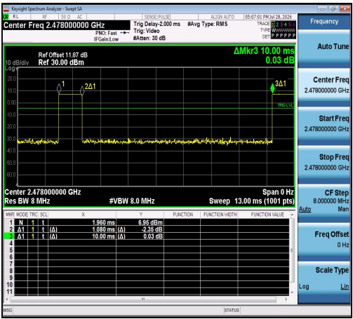
NTNV-LE_2M-Ant1-2478
