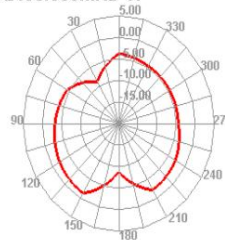
2450.000MHz E2
