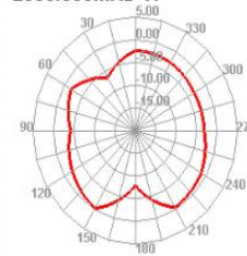
2500.000MHz H
