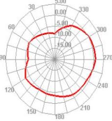
2400.000MHz E2
