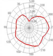
2500.000MHz H
