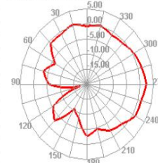
2500.000MHz E2
