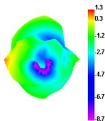
2400.000MHz E1
