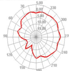
2450.000MHz E2
