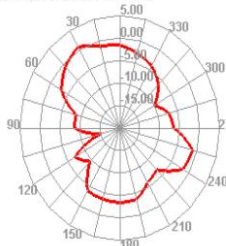
2450.000MHz E1
