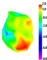
2400.000MHz E1
