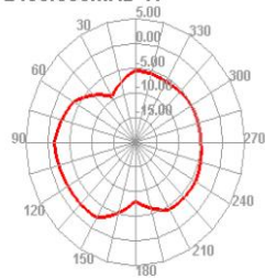
2400.000MHz E2
