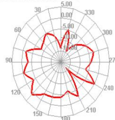
2450.000MHz E2
