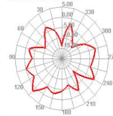
2500.000MHz E2
