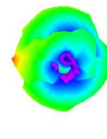
2500.000MHz E1
