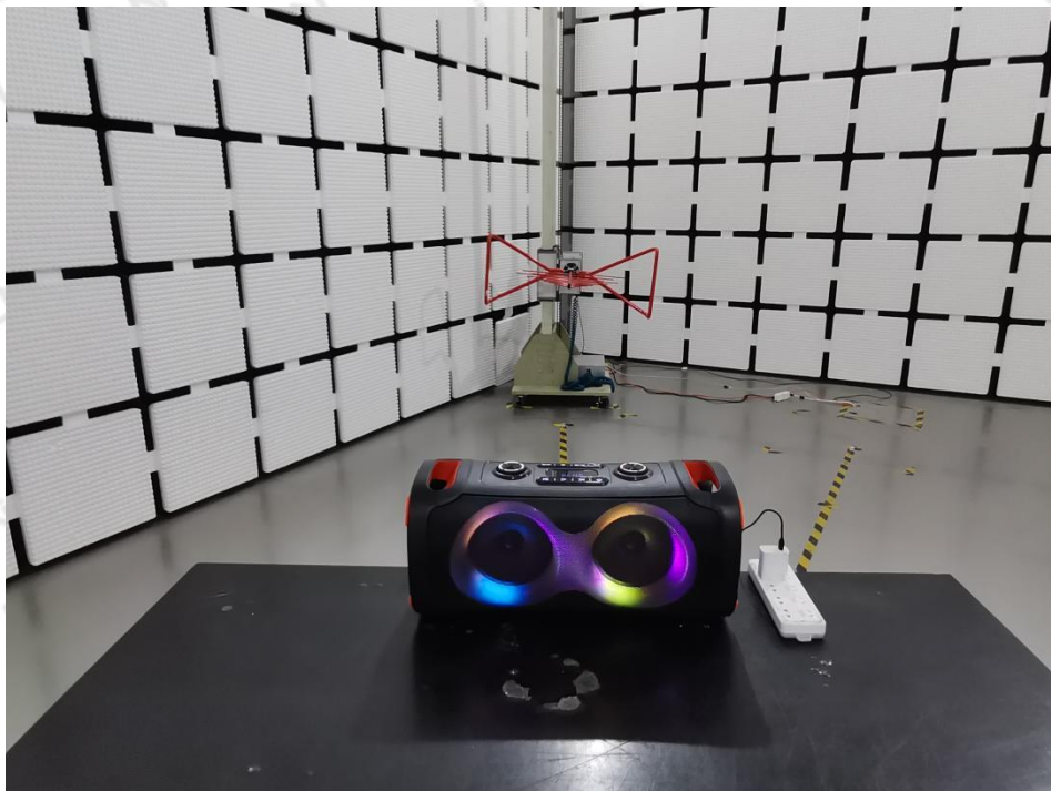
30MHz-1000MHz
