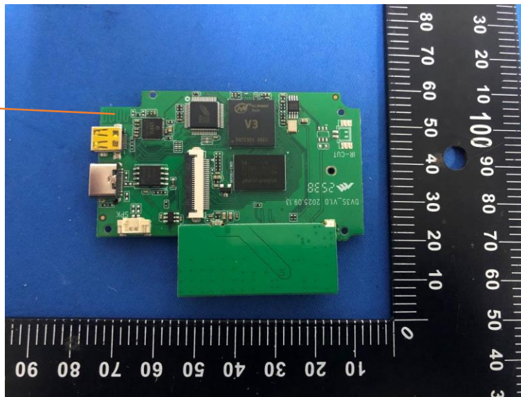
2.4GWIFI ANT
