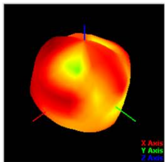
WIFI 5.8G天线3D图
