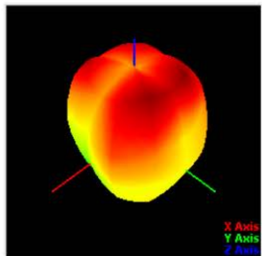
WIFI 2.4G天线3D图
