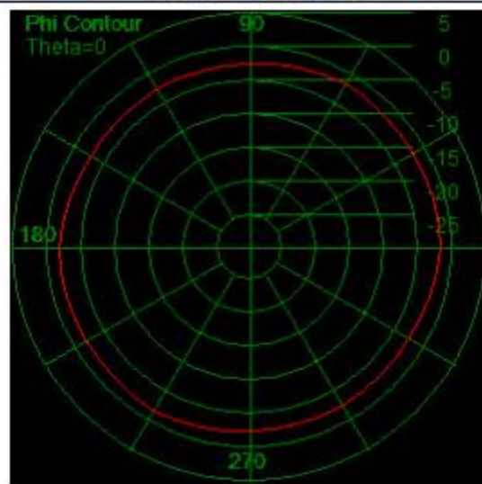
天线2D图H面
