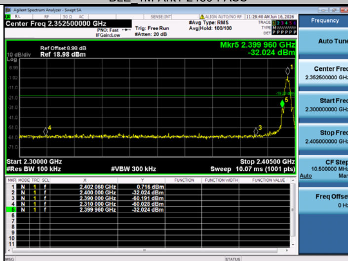
BLE 2M-Ant1-2402-PASS
