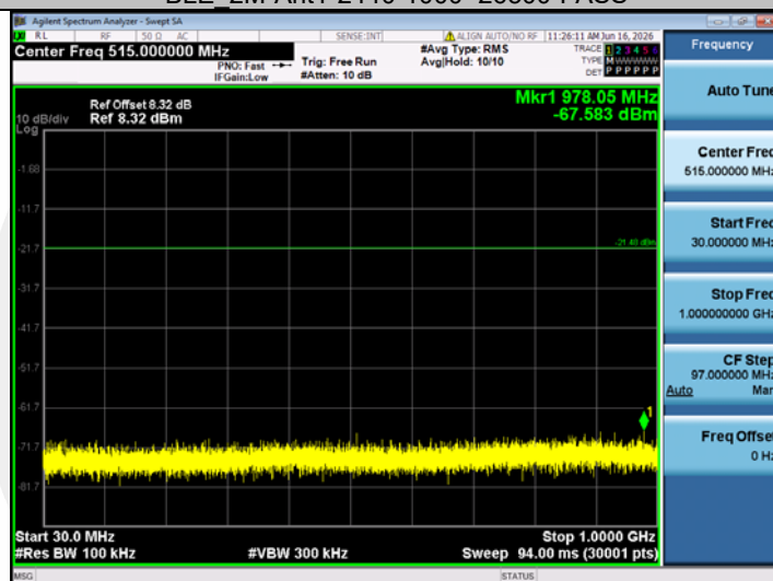
BLE_2M-Ant1-2480-30~1000-PASS
