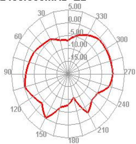
2400.000MHz E2
