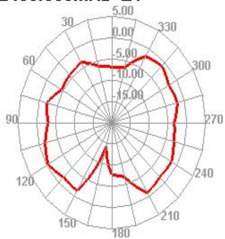
2400.000MHz E1
