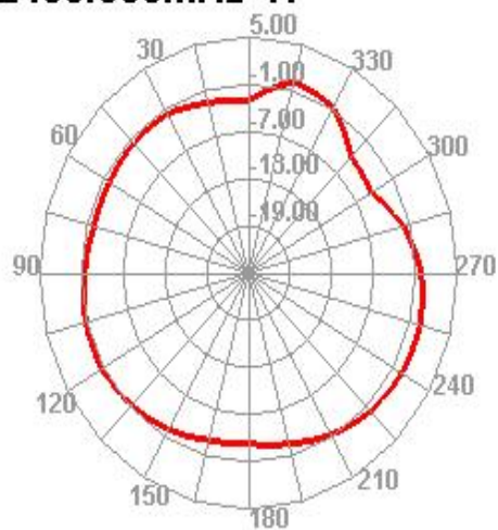
2400.000MHz H
