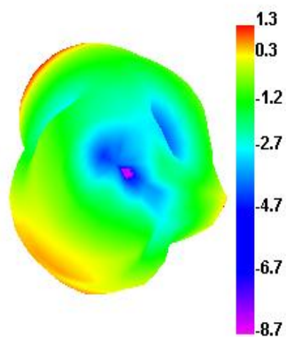
2400.000MHz H
