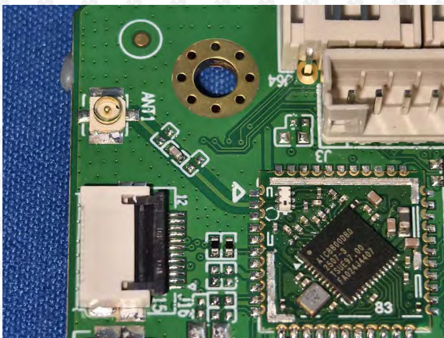
EUT Photo 12
