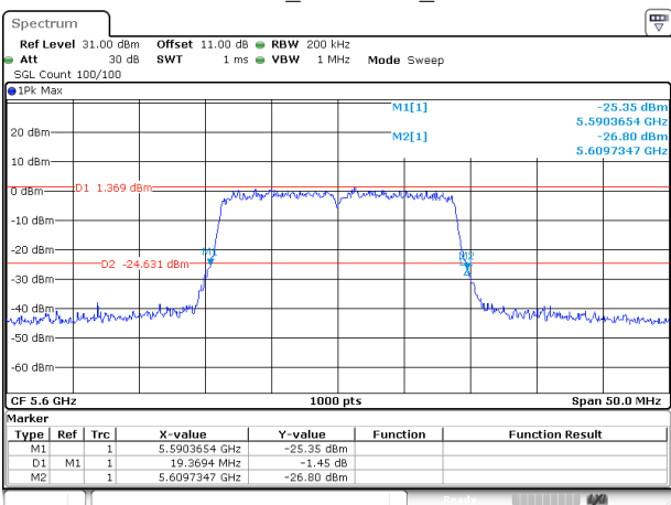
802.11ac20_5600MHz_Chain 0
