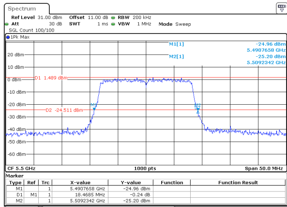
802.11a_5500MHz_Chain 1
