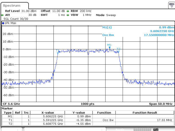
802.11ac20_5600MHz_Chain 0
