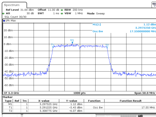
802.11ac20_5300MHz_Chain 1
