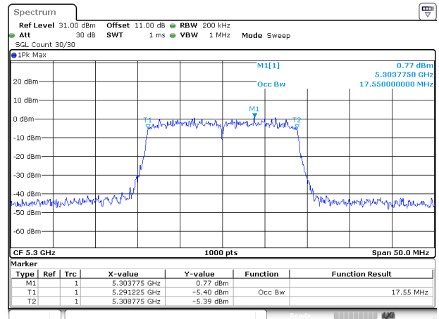
802.11ac20_5300MHz_Chain 0
