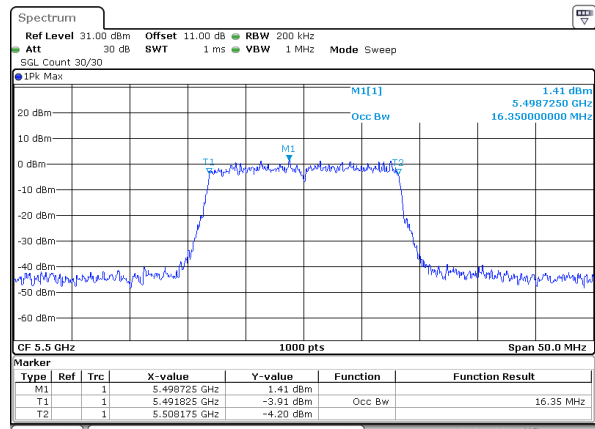
802.11a_5500MHz_Chain 1
