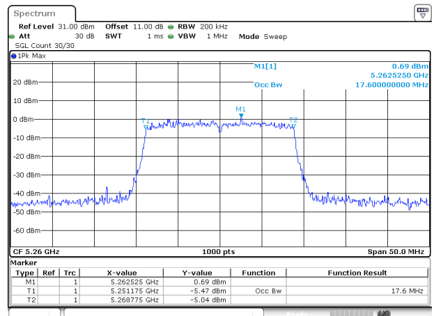
802.11ac20_5260MHz_Chain 1
