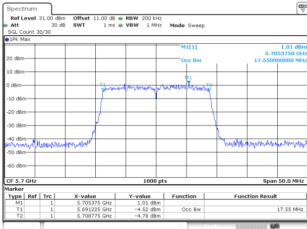
802.11ac20_5700MHz_Chain 0
