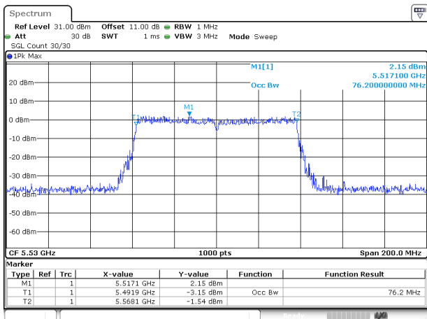
802.11ac80_5530MHz_Chain 0
