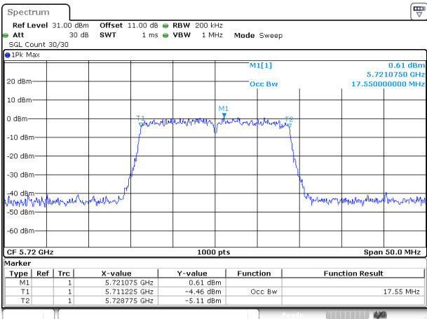
802.11ac20_5720MHz_Chain 0
