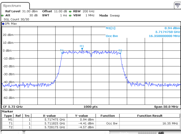
802.11a_5720MHz_Chain 1
