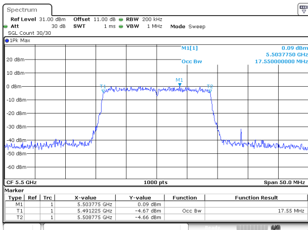
802.11ac20_5500MHz_Chain 0
