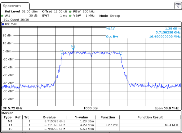
802.11a_5720MHz_Chain 0
