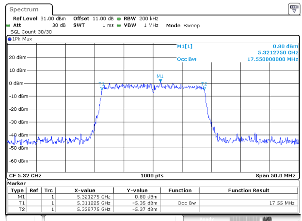
802.11ac20_5320MHz_Chain 1
