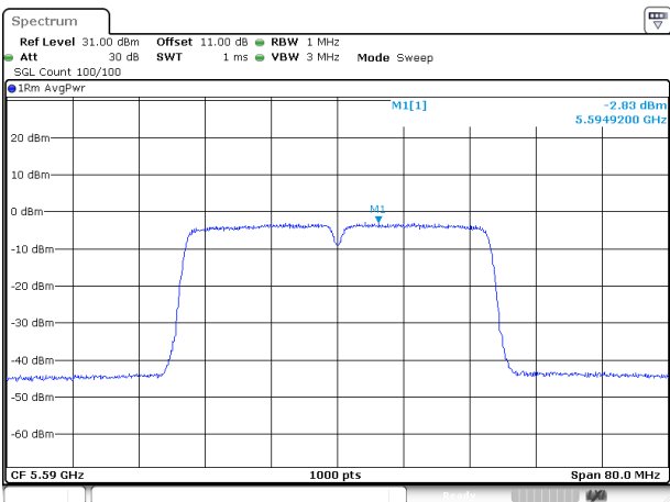
802.11ac40_5590MHz_Chain 0
