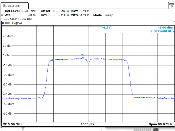
802.11ac40_5590MHz_Chain 1
