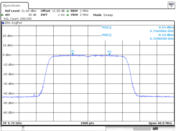
802.11ac20_5720MHz_Chain 0
