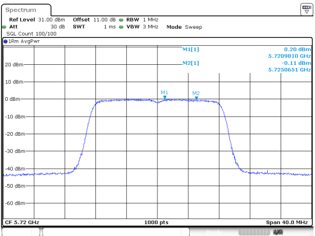
802.11a_5720MHz_Chain 1
