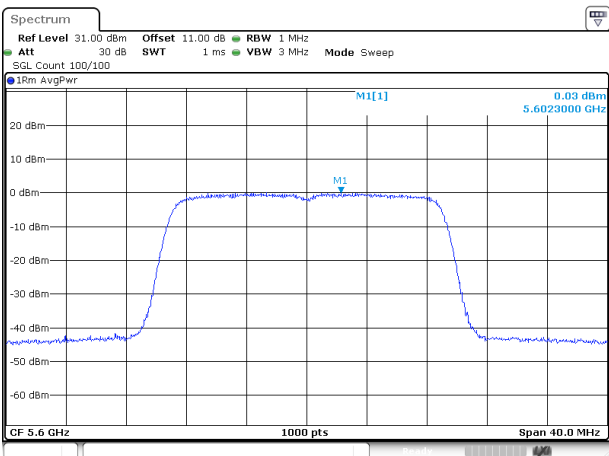
802.11ac20_5600MHz_Chain 1
