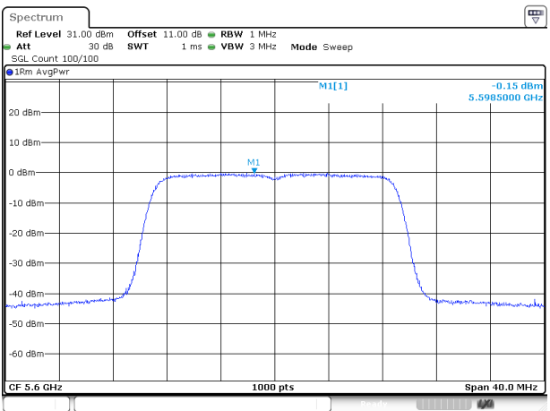
802.11ac20_5600MHz_Chain 0
