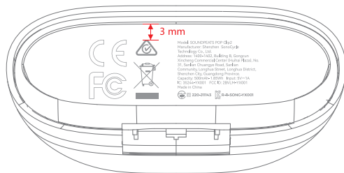
耳机盒上盖
