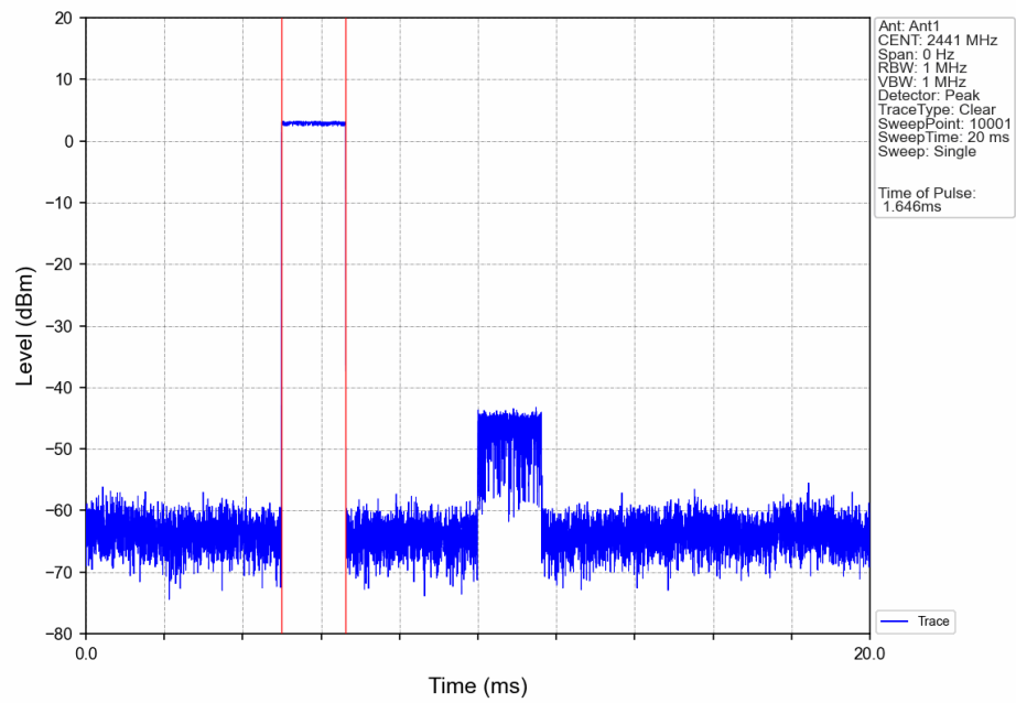
GFSK_DH3_HOPP_Ant1_NTNV
