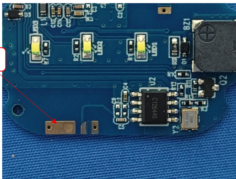
BLE Antenna
