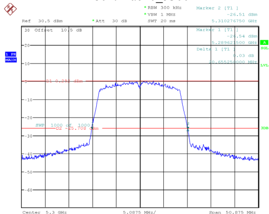
802.11ac20_5300MHz
