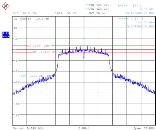
802.11ac20_5745MHz
