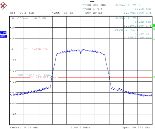
802.11ac20_5260MHz
