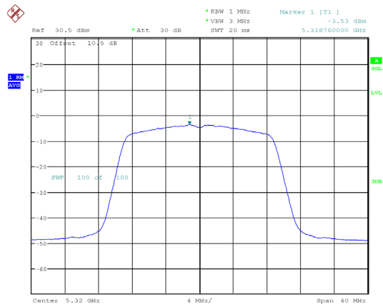
802.11ac20_5320MHz
