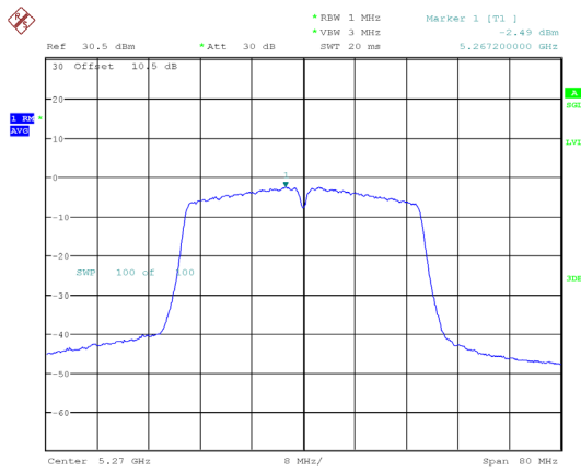
802.11ac40_5270MHz
