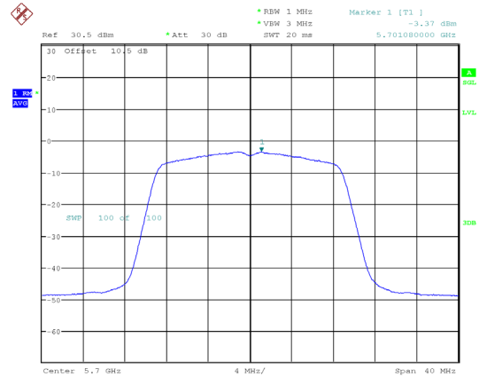
802.11ac20_5700MHz
