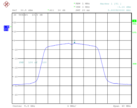
802.11ac20_5600MHz
