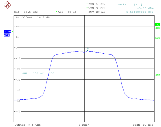
802.11ac20_5500MHz
