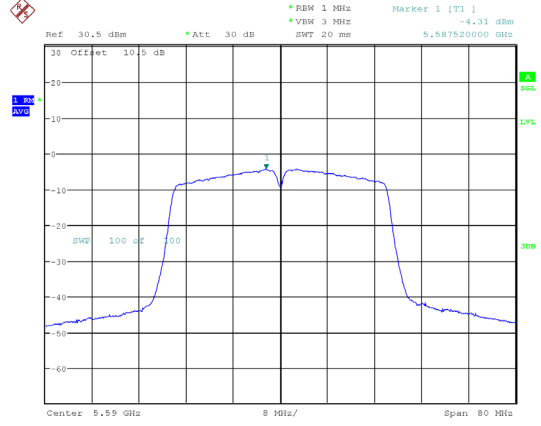
802.11ac40_5590MHz
