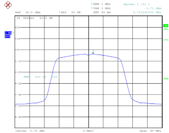
802.11ac20_5720MHz
