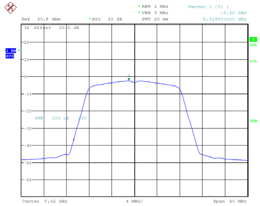
802.11a_5320MHz
