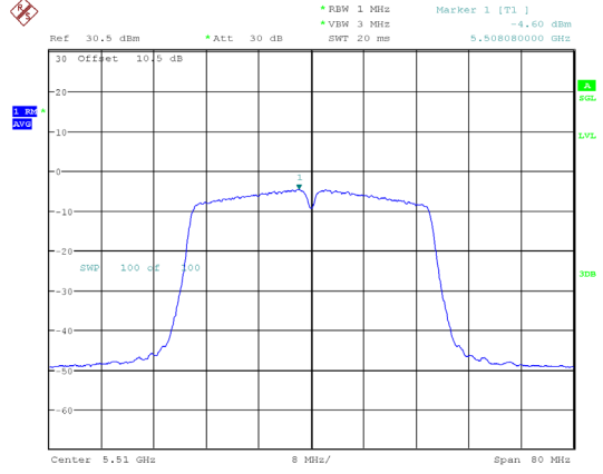
802.11ac40_5510MHz
