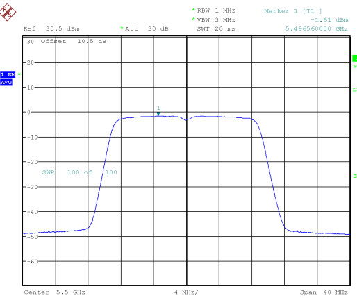
802.11ac20_5500MHz
