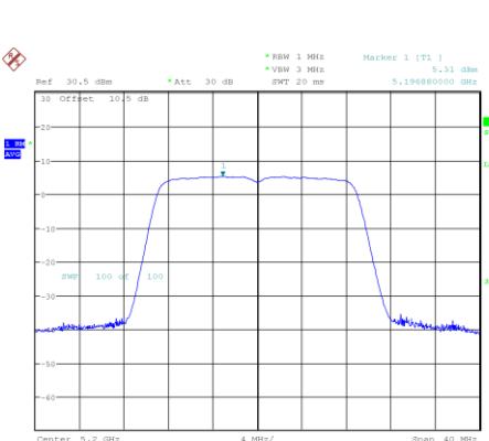
802.11ac20_5200MHz
