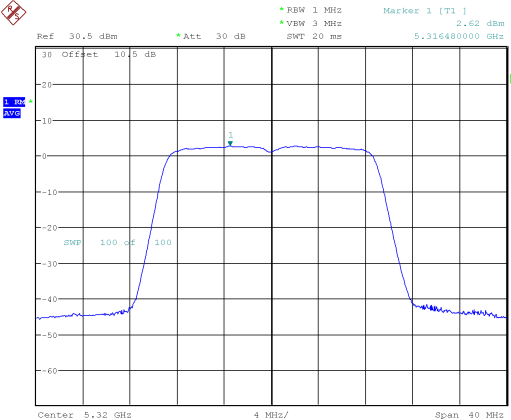
802.11ac20_5320MHz
