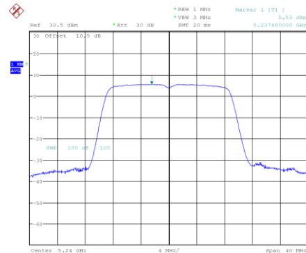
802.11ac20_5240MHz
