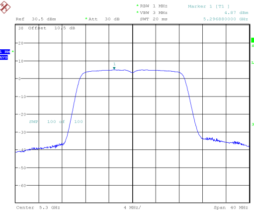
802.11ac20_5300MHz
