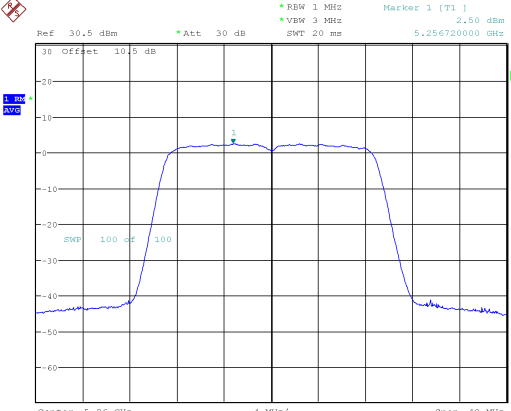
802.11ac20_5260MHz
