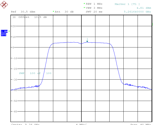
802.11ac20_5260MHz
