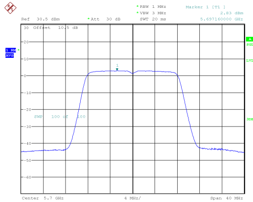
802.11a_5700MHz
