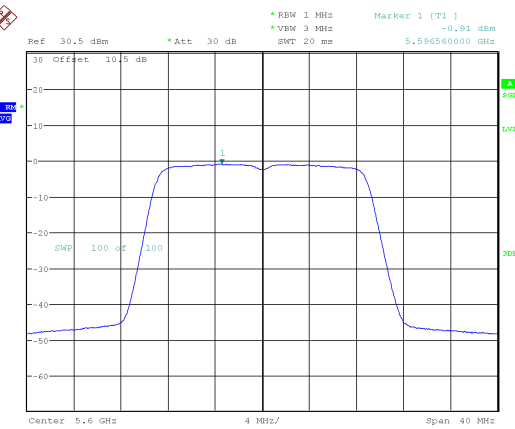
802.11ac20_5600MHz
