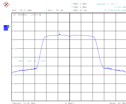
802.11ac20_5180MHz
