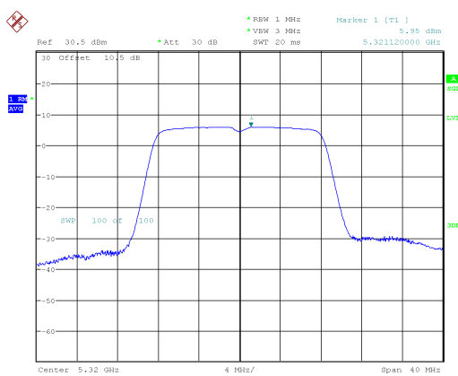
802.11a_5320MHz
