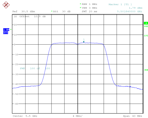
802.11a_5500MHz
