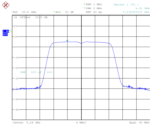
802.11ac20_5240MHz
