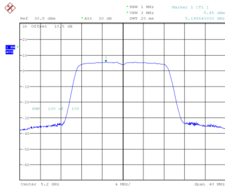
802.11ac20_5200MHz
