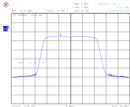
802.11ac20_5180MHz
