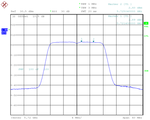
802.11a_5720MHz
