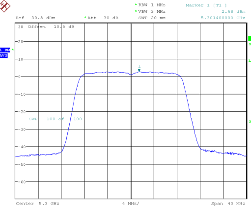
802.11ac20_5300MHz
