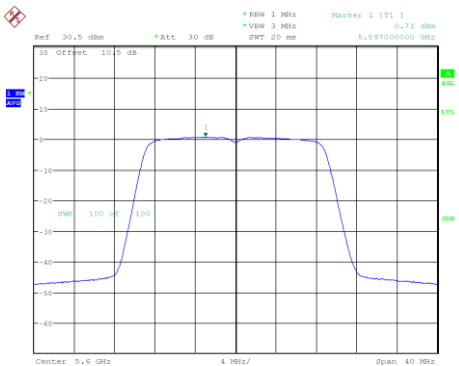
802.11ac20_5600MHz
