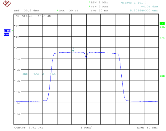
802.11ac40_5510MHz
