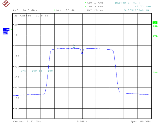
802.11ac40_5710MHz
