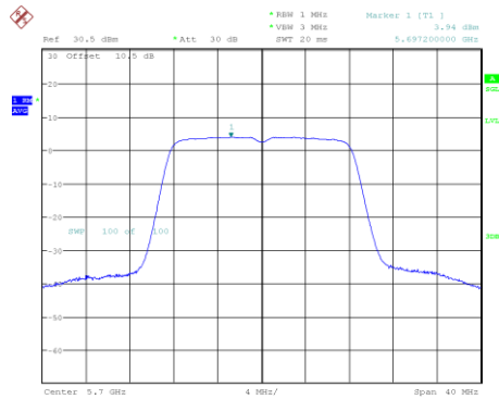
802.11a_5700MHz
