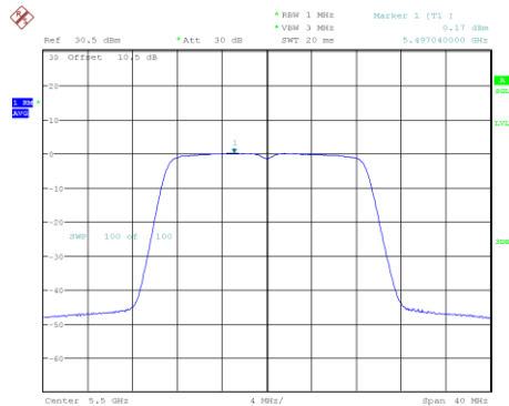
802.11ac20_5500MHz
