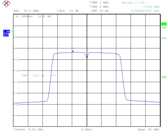
802.11ac40_5590MHz
