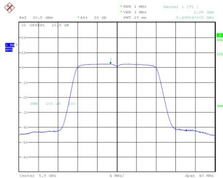
802.11a_5500MHz
