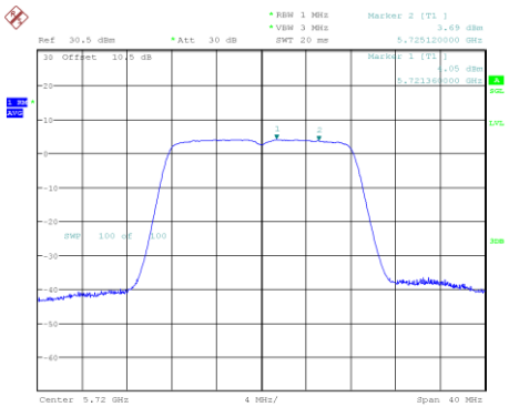
802.11a_5720MHz
