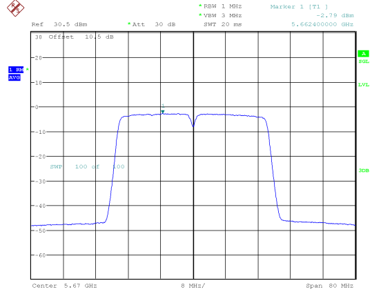
802.11ac40_5670MHz
