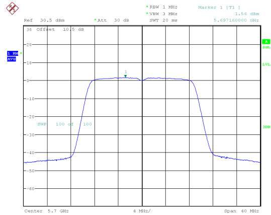
802.11ac20_5700MHz
