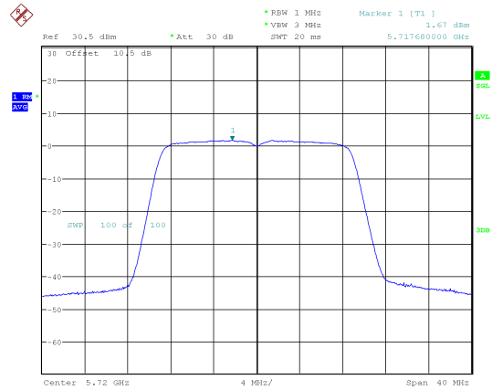
802.11ac20_5720MHz
