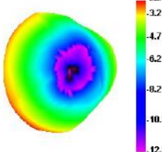
6000.000MHz
