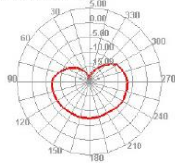
5000.000MHz H
