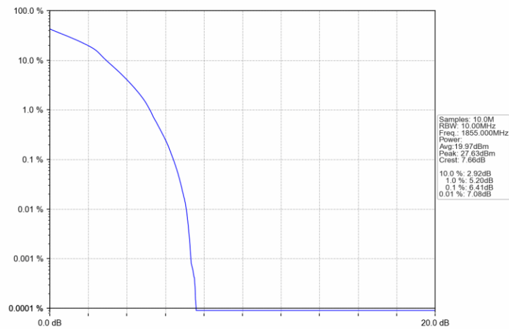
Band2_10MHz_16QAM_LCH_1855MHz_RB_27_0_NTNV
