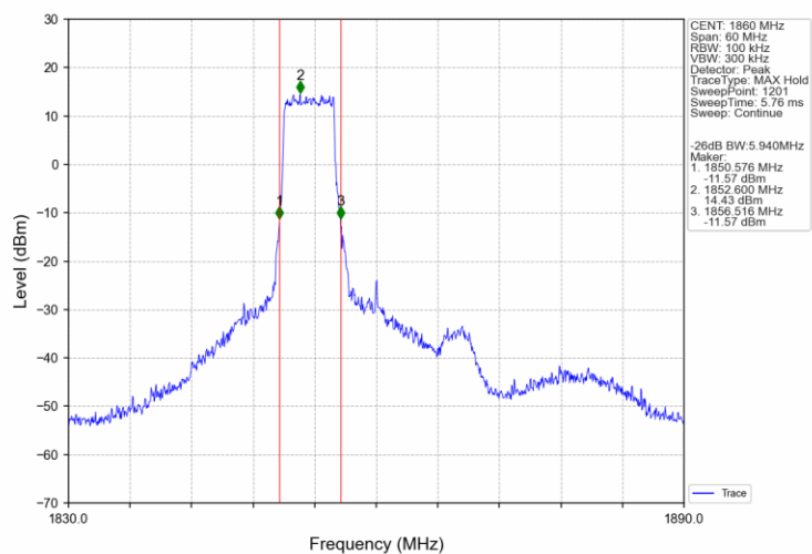
Band2_20MHz_16QAM_LCH_1860MHz_RB_27_0_NTNV
