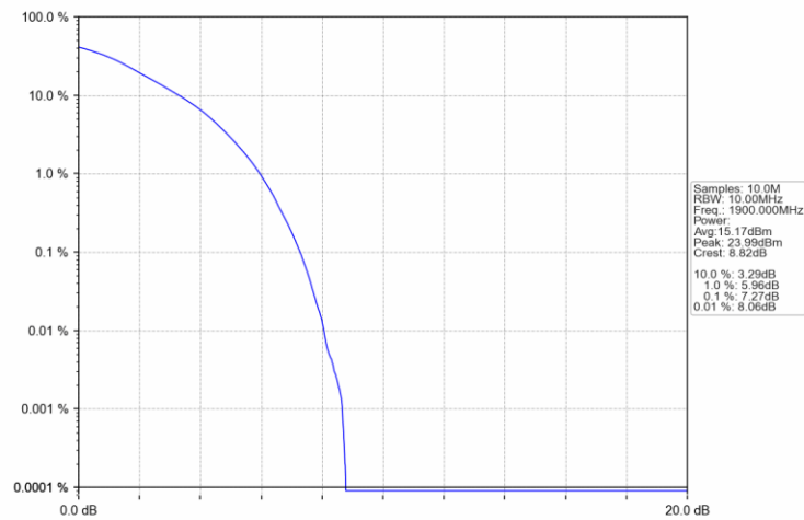
Band2_20MHz_16QAM_HCH_1900MHz_RB_27_73_NTNV
