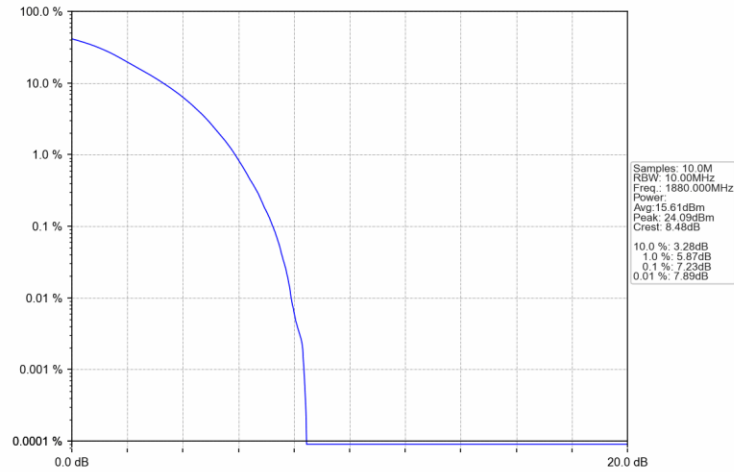
Band2_20MHz_16QAM_MCH_1880MHz_RB_27_0_NTNV
