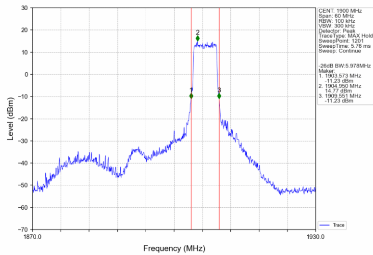
Band2_20MHz_16QAM_HCH_1900MHz_RB_27_73_NTNV
