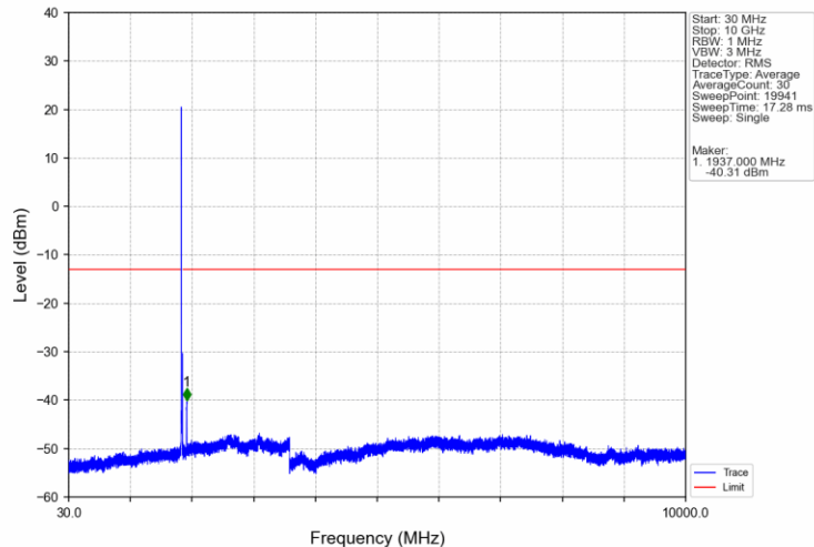
Band2_10MHz_QPSK_LCH_1855MHz_RB_1_0_NTNV
