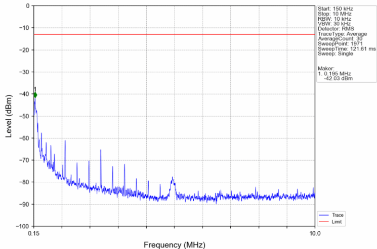
Band4_15MHz_QPSK_LCH_1717.5MHz_RB_1_0_NTNV
